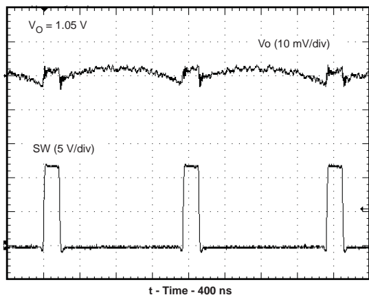
図 15. 出力電圧リップル ( I_O = 2A )
