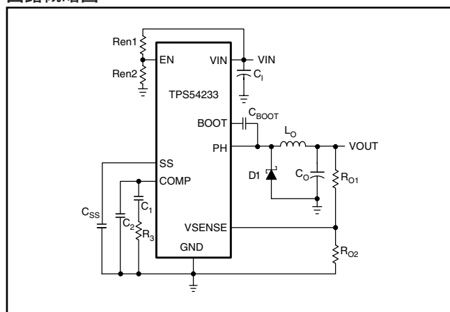
回路概略図
