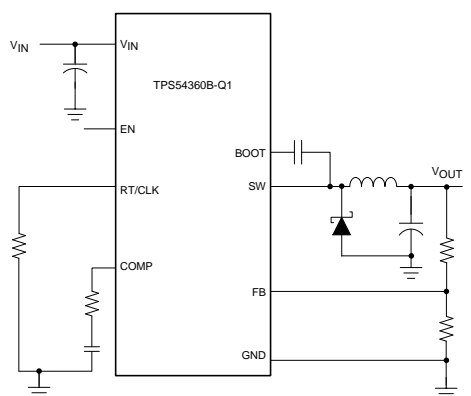
概略回路図
