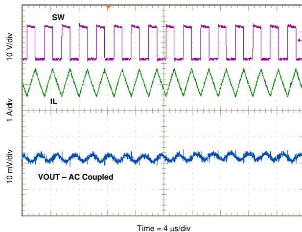
8-10. Output Ripple CCM
