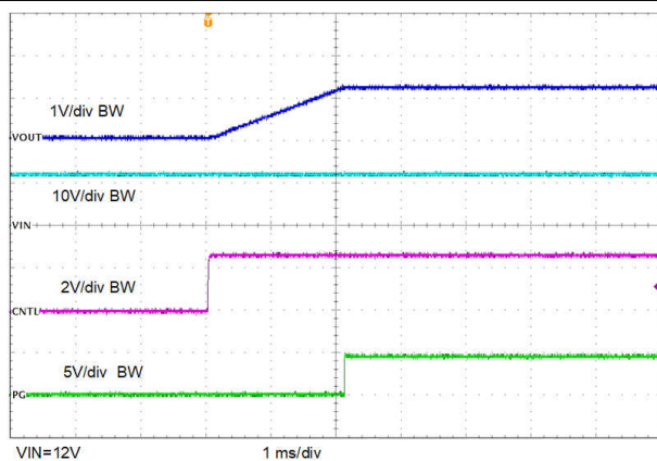
図 8-12. 制御からのスタートアップ、0A 負荷
