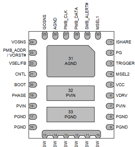
図 4-2. VBD 33 ピン WQFN パッケージ (底面図)
