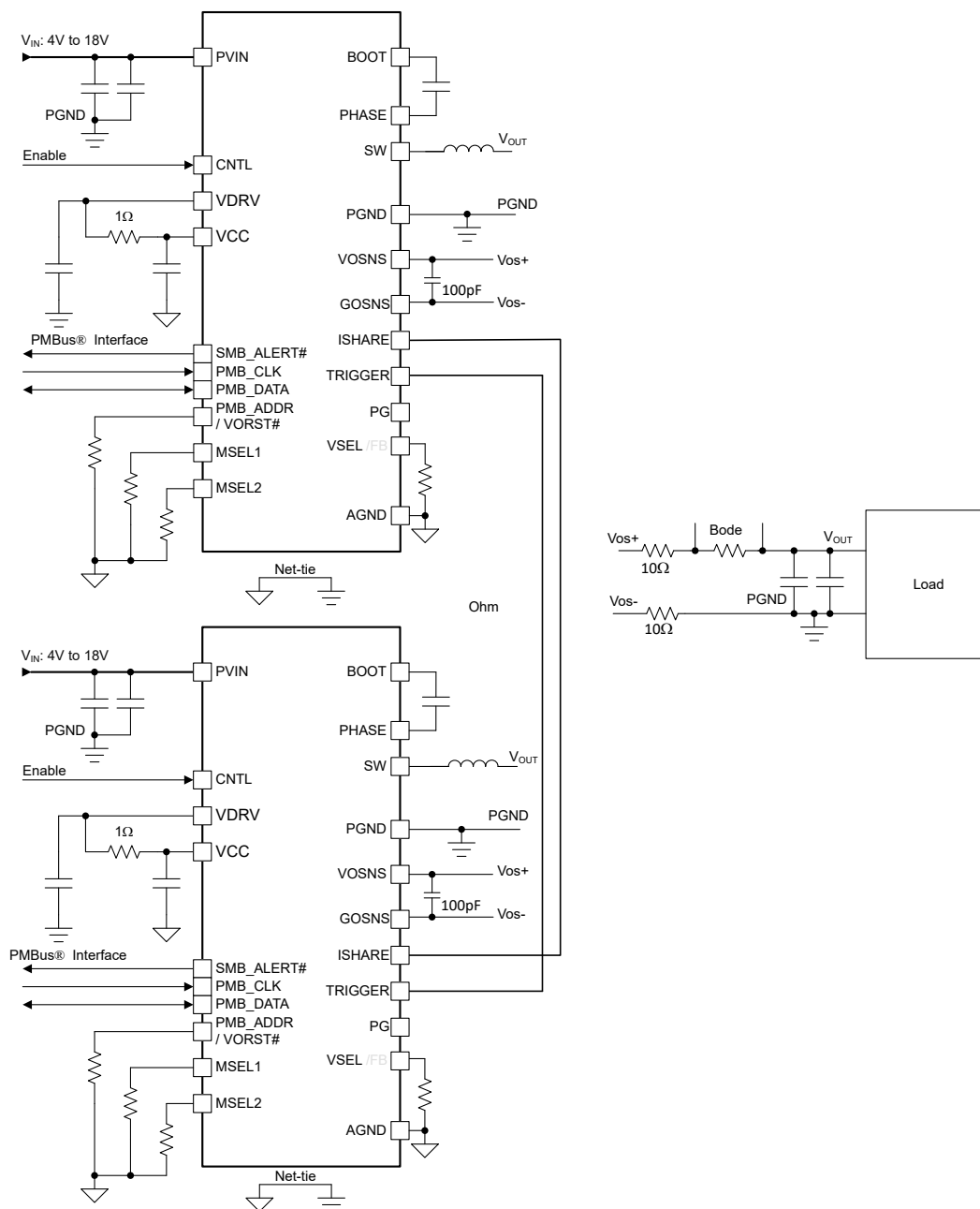
図 6-7. 2 相構成の内部分圧器
