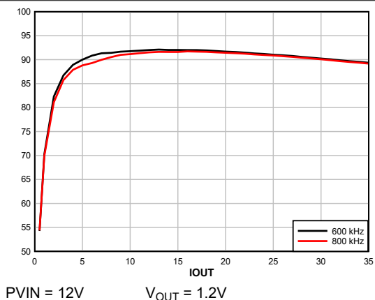
図 8-6. 効率、FCCM、外部 5V バイアス
