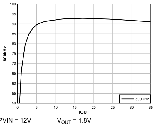
図 8-8. 効率、FCCM、内部 LDO
