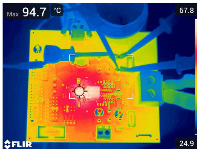
図 8-19. 熱画像、800kHz FCCM、35A 負荷
