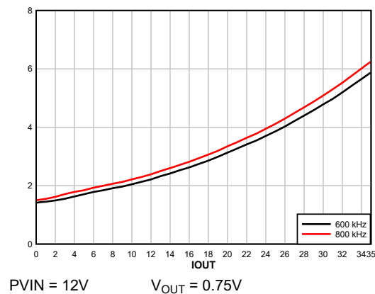
図 8-3. 消費電力、FCCM、内部 LDO
