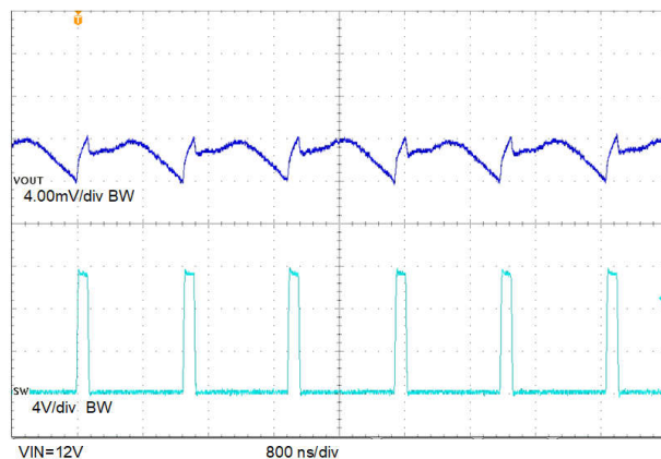
図 8-16. 出力電圧リップル、800kHz FCCM、17.5A 負荷
