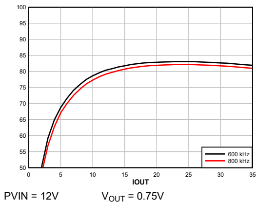
図 8-2. 効率、FCCM、内部 LDO
