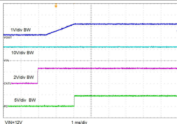
図 8-13. プリバイアス出力による制御からのスタートアップ
