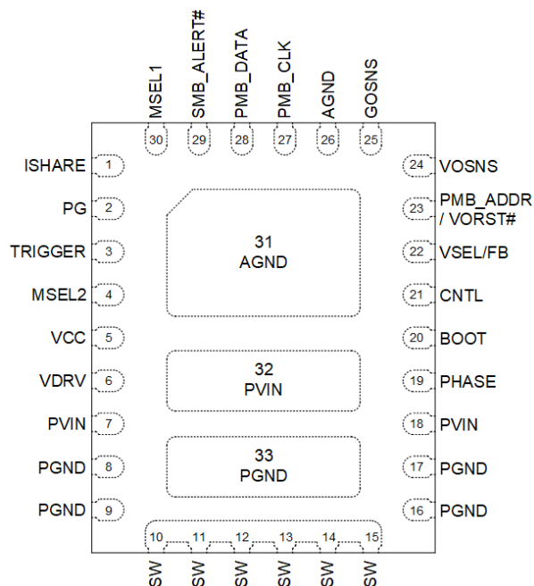
図 4-1. VBD 33 ピン WQFN パッケージ (上面図)
