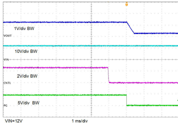
図 8-14. 制御からのシャットダウン、0A 負荷
