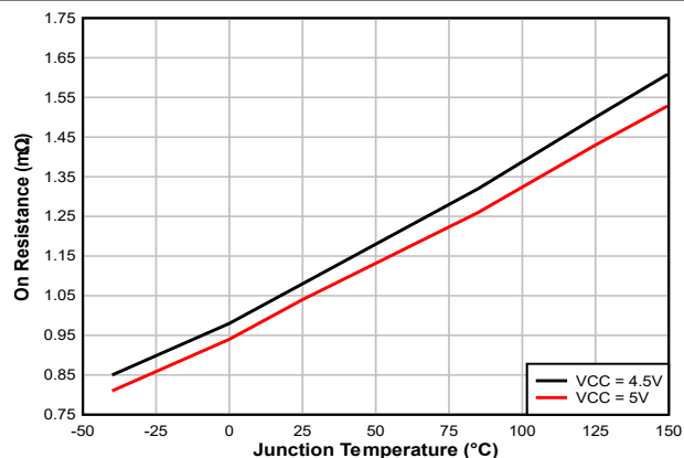
図 5-4. ローサイド MOSFET オン抵抗 ( R_{DS(on)} ) と接合部温度との関係
