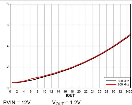
図 8-7. 消費電力、FCCM、外部 5V バイアス
