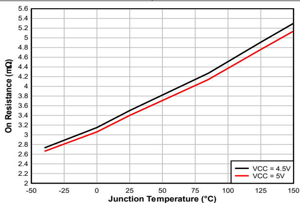
図 5-5. ハイサイド MOSFET オン抵抗 ( R_{DS(on)} ) と接合部温度との関係
