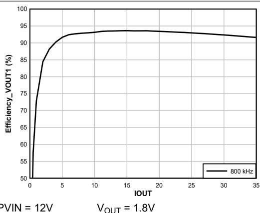
図 8-10. 効率、FCCM、外部 5V バイアス
