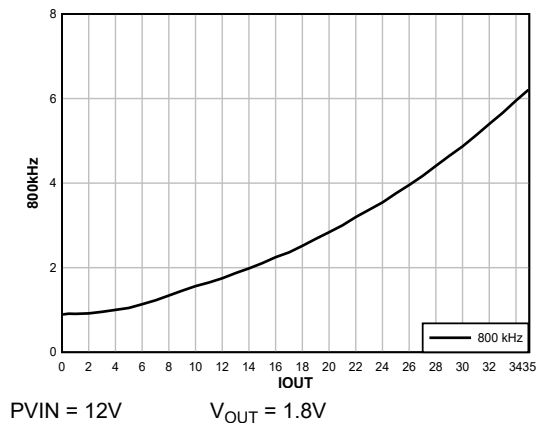
図 8-9. 消費電力、FCCM、内部 LDO
