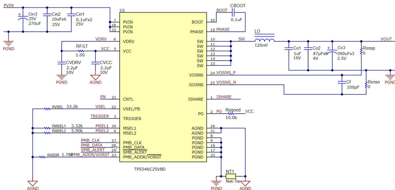
図 8-1. 1.2V、35A 出力のアプリケーション
