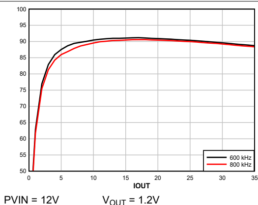
図 8-4. 効率、FCCM、内部 LDO
