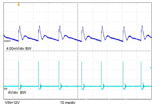
図 8-17. 出力電圧リップル、1.2V Vout、800kHz DCM、無負荷
