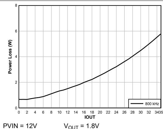
図 8-11. 消費電力、FCCM、外部 5V バイアス
