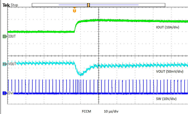
6-11. Load Transient
