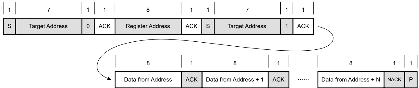
図 6-14. Multibyte Read
