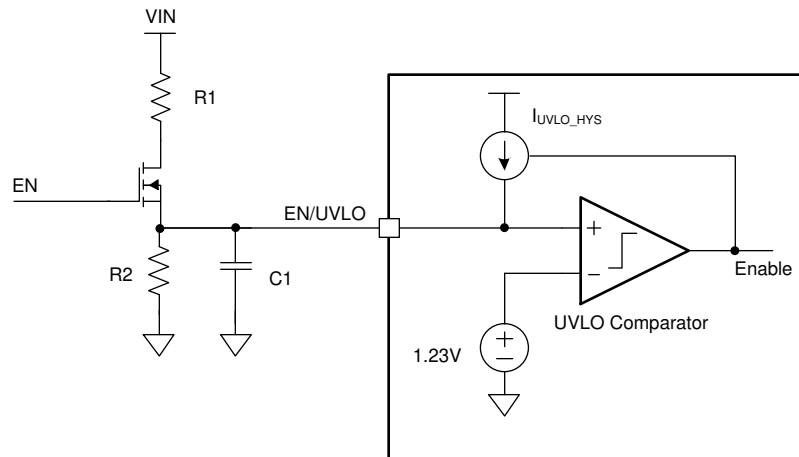
図 6-2. Logic Enable and Programmable UVLO
