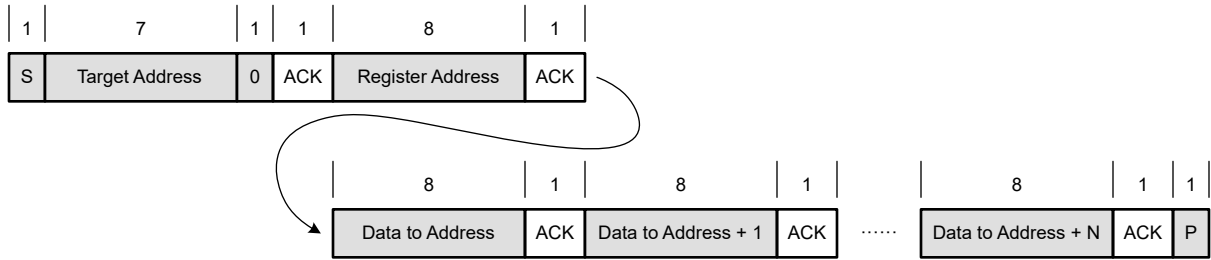
図 6-13. Multibyte Write
