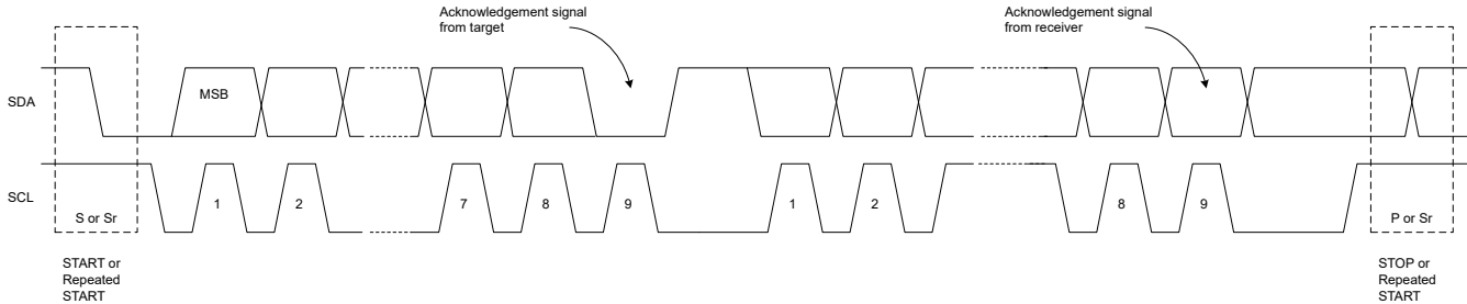
6-9. Byte Format
