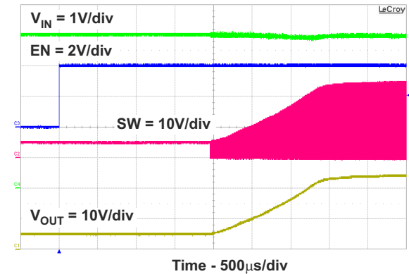
9-8. Start Up
