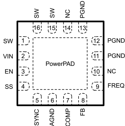
図 6-1. 16-Pin WQFN RTE Package (Top View)
