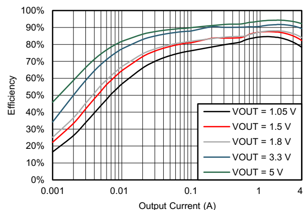
TPS564201の効率
