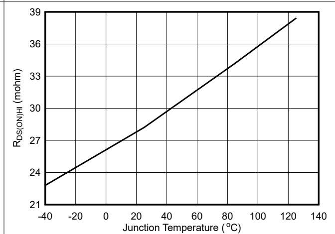
图 6-6. High-Side R_{DS(ON)}
