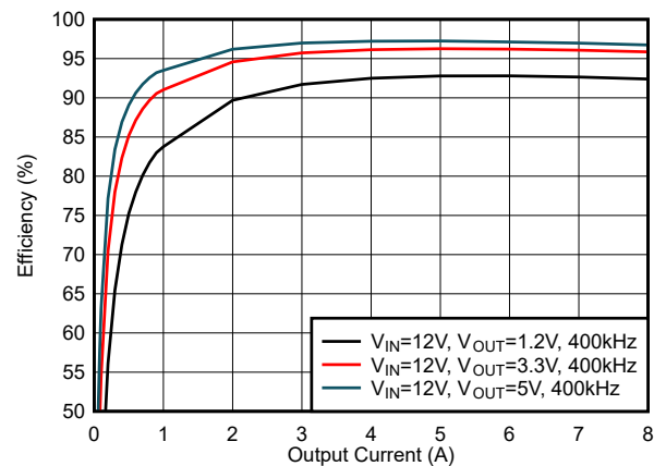
効率、FCCM モード
