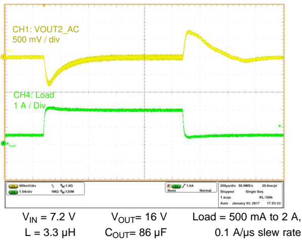
30. Load Transient
