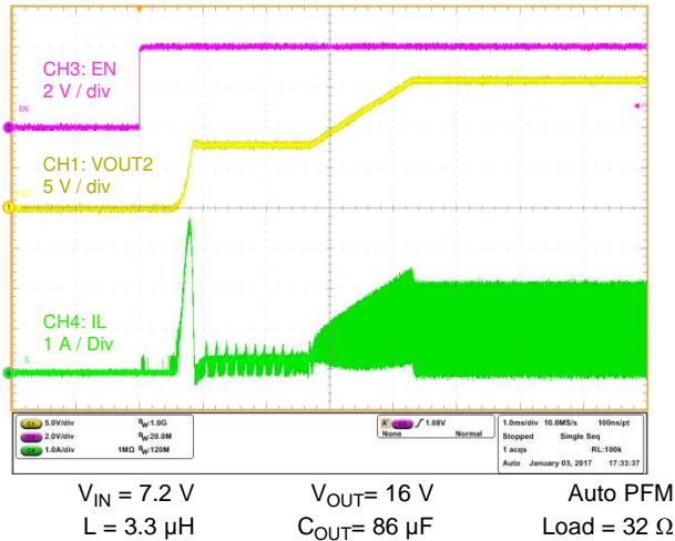
28. Startup by EN
