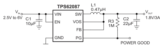
代表的なアプリケーション回路図
