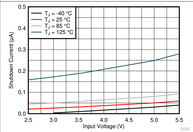
图 6-4. Shutdown Current
