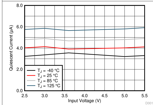
图 6-3. Quiescent Current
