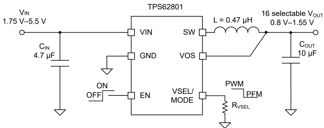
図 8-48. TPS62801 可変 V_{OUT} アプリケーション回路
