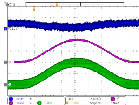
TPS62801 V_{OUT} = 1.2\text{ V} VSEL/MODE = VIN (起動後) 強制 PWM モード I_{OUT} = 1\text{ mA} \sim 1\text{ A} , 1kHz
