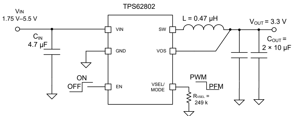
図 8-49. TPS62802 可変 3.3V V_{OUT} アプリケーション回路
