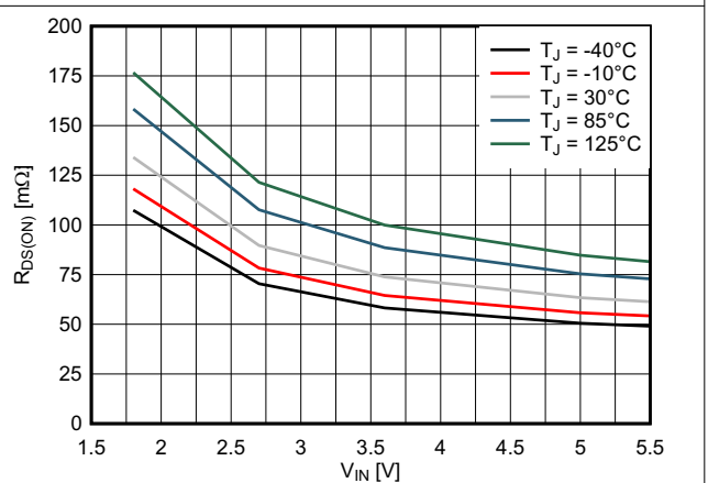
図 6-6. ローサイドスイッチのドレインソース抵抗、 R_{DS(ON)}
