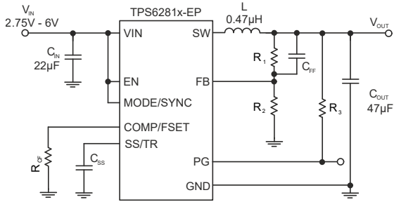
概略回路図
