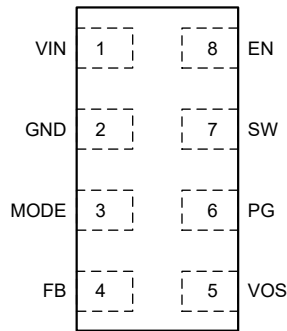
図 5-1. RZE Package 8-Pin WQFN Top View
