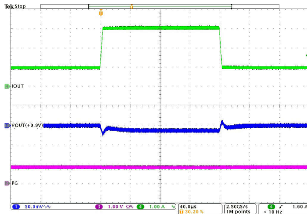
図 8-33. Load Transient
