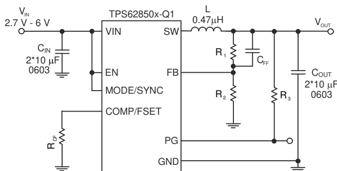
概略回路図
