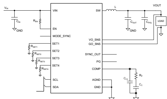
TPS6289x-Q1 の概略回路図
