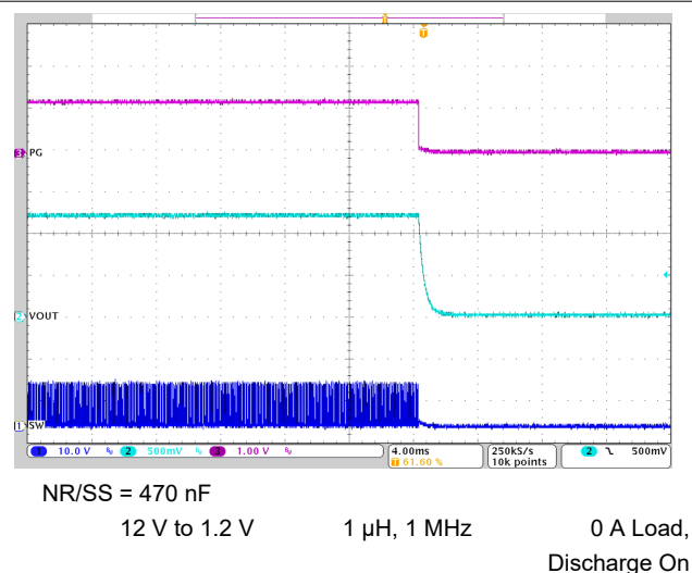
図 7-11. Shutdown
