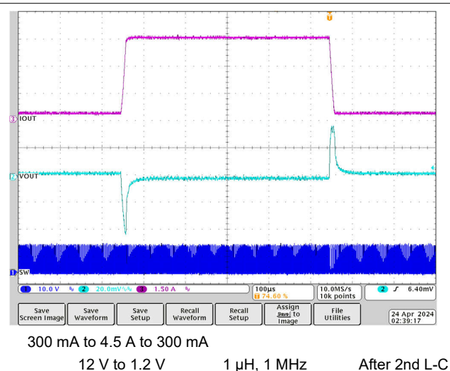
図 7-13. Load Transient
