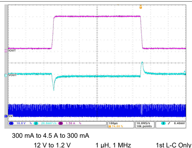
図 7-12. Load Transient
