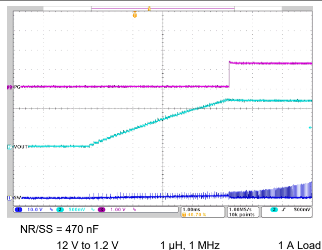
図 7-10. Start-up
