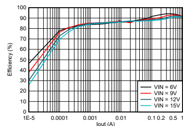
効率と出力電流との関係 V_{OUT} = 3.3V (2.5MHz 自動 PFM/PWM)
