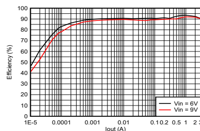
効率と出力電流との関係 (2.5MHz、1 \mu H、自動 PFM または PWM で V_O = 3.3V )
