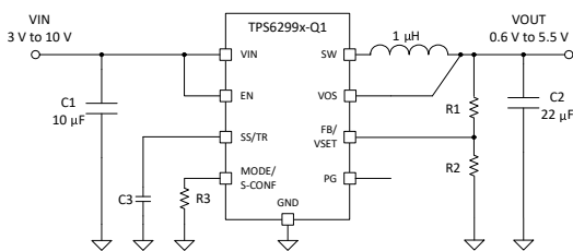
簡略回路図
