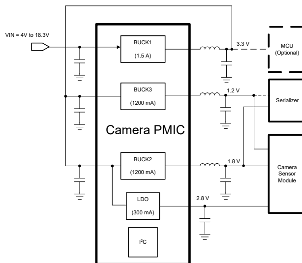
TPS650350-Q1 アプリケーション回路
