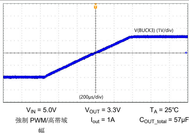
図 7-4. Buck3 ランプ
