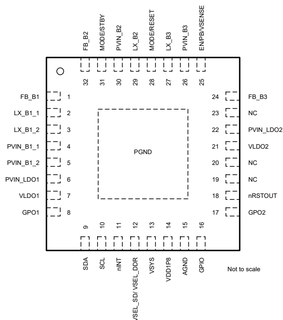
図 4-1. TPS65215-Q1 RHB パッケージ、32 ピン QFN (上面図)
