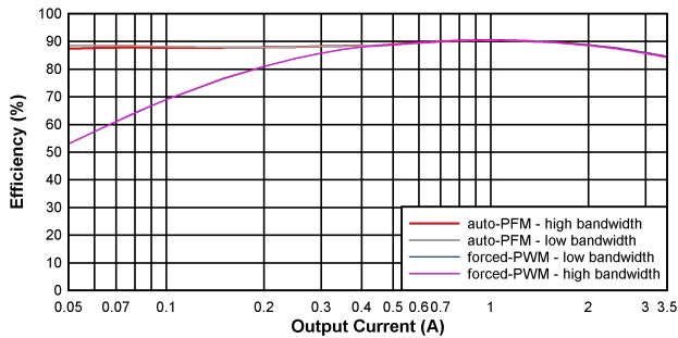
図 6-1. 効率 BUCK1
