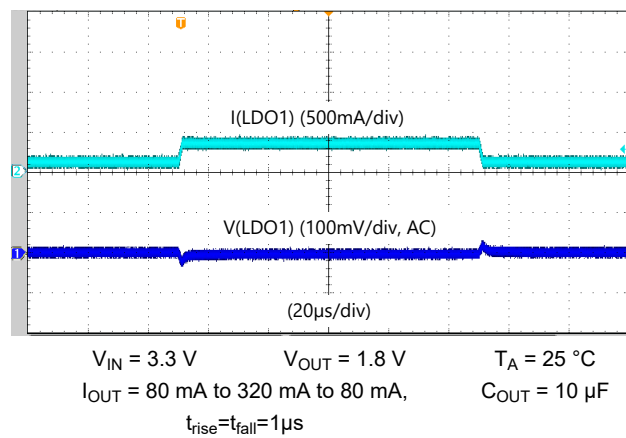
図 6-6. LDO1 Load-step response
