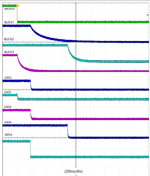
8-9. LDOs Discharge
