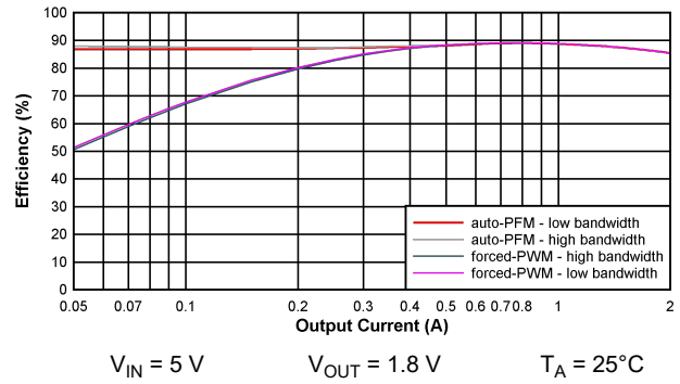
図 6-2. Efficiency BUCK23
