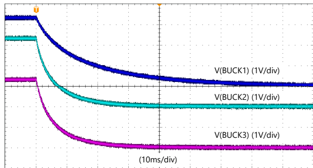
V_{IN} = 5.0V V_{OUT} = 3.3V T_A = 25^\circ C 強制 PWM/高帯域 幅 無負荷 C_{OUT\_total} = 57\mu F
