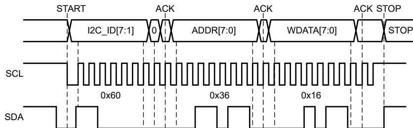
图 7-8. I 2 C Write Cycle without CRC
