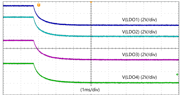
8-9. LDOs Discharge
