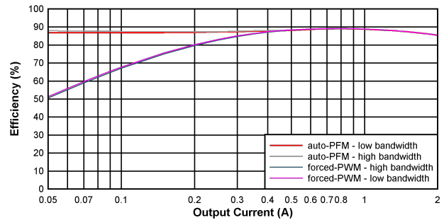
図 6-2. 効率 BUCK23
