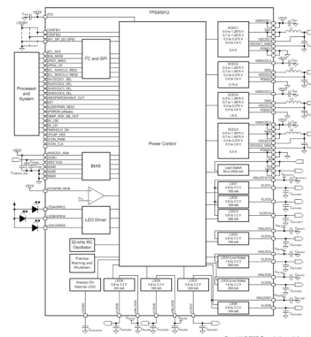
概略回路図
