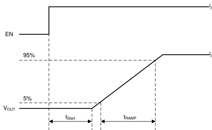
図 8-1. Soft Start
