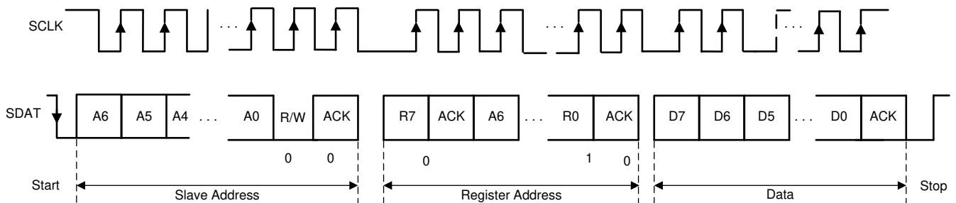
图 8-22. Bus Protocol
