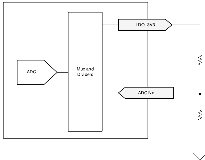
8-17. ADCINx Resistor Divider
