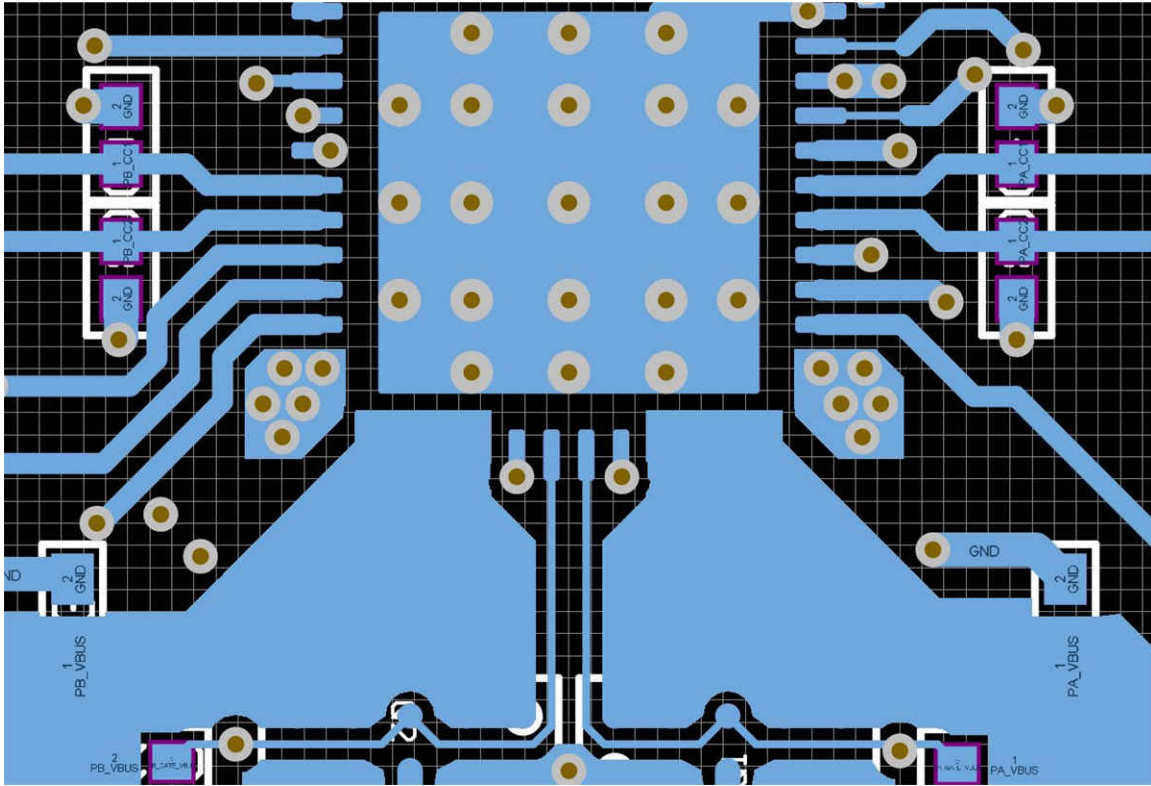
✎ 11-6. VBUS1 and VBUS2 Copper Pours and Via Placement (Top)
