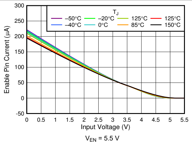
6-22. I_{EN} vs V_{IN}
