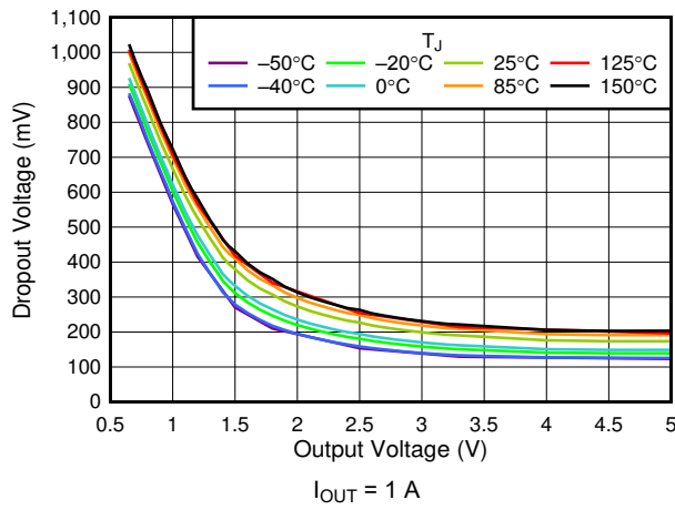
6-7. V_{DO} vs V_{OUT}
