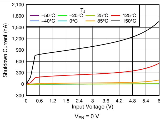
6-9. I_{SHDN} vs V_{IN}
