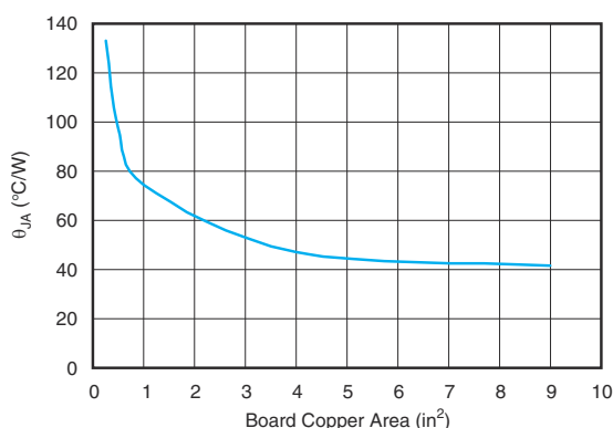
図 7-4. R_{\theta JA} vs Board Size
