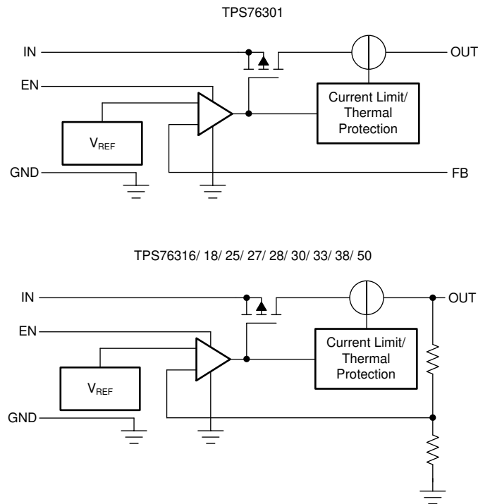
図 6-1. 機能ブロック図 (従来チップ)
