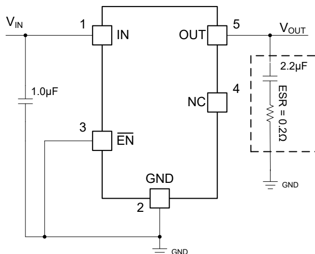
代表的なアプリケーション回路
