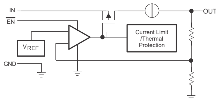
图 6-2. TPS769-Q1 Functional Block Diagram (Legacy Chip)
