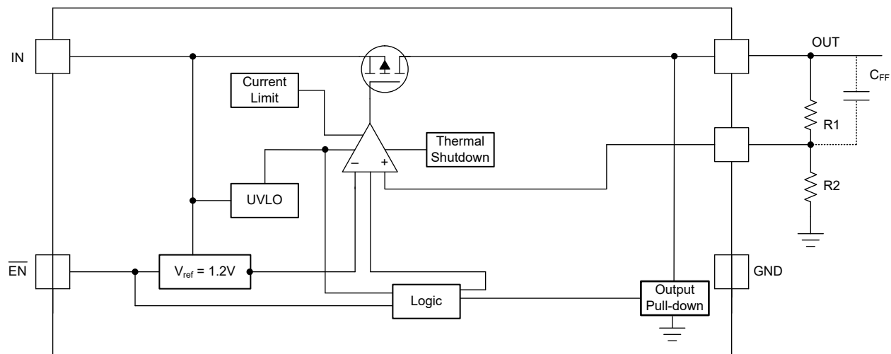
图 6-3. TPS76901-Q1 Functional Block Diagram (New Chip)
