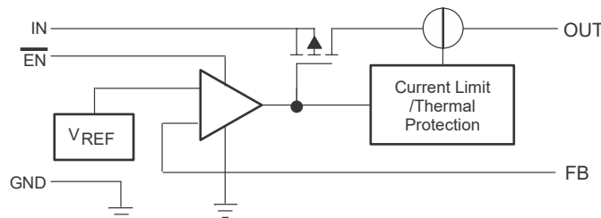
图 6-1. TPS76901-Q1 Functional Block Diagram (Legacy Chip)
