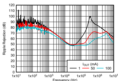
TPS76933-Q1 PSRR と出力電流との関係 (新しいチップ)
