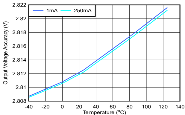
図 6-4. TPS794 出力電圧と接合部温度との関係
