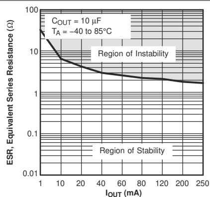
図 6-34. TPS794 標準安定動作領域等価直列抵抗 (ESR) と出力電流との関係
