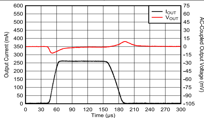
図 8-7. TPS794 の負荷過渡応答
