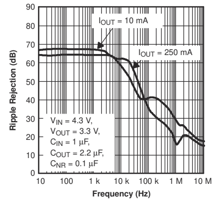
図 6-20. TPS794 リップル除去と電流との関係
