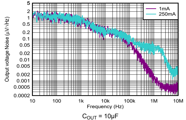
図 6-10. TPS794 出力スペクトル ノイズ密度と周波数との関係
