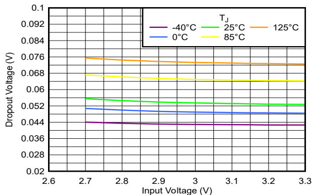
図 6-32. TPS794 ドロップアウト電圧 対 入力電圧
