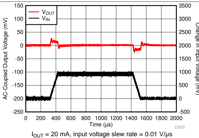
20. V_{IN} Transient
