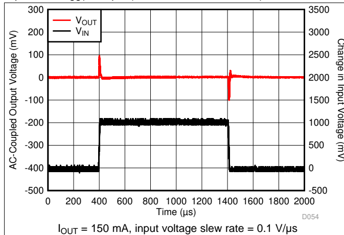
19. V_{IN} Transient
