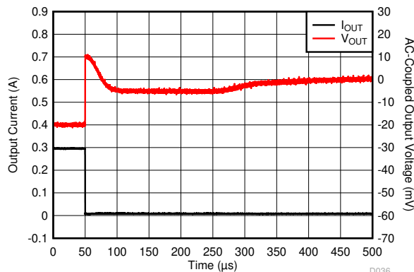
图 5-39. Load Transient
