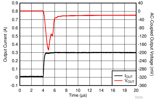
图 5-38. Load Transient
