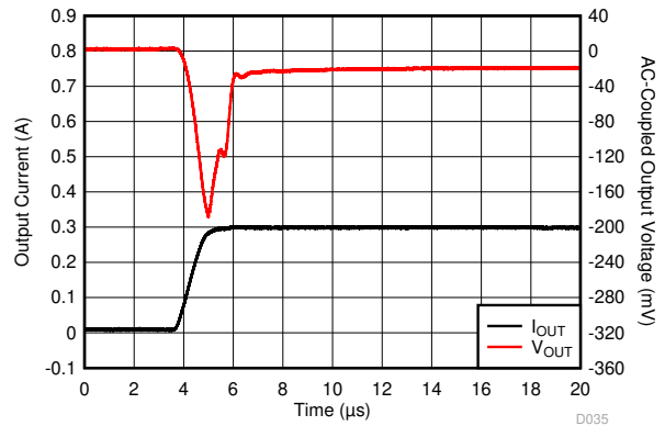
图 5-38. Load Transient
