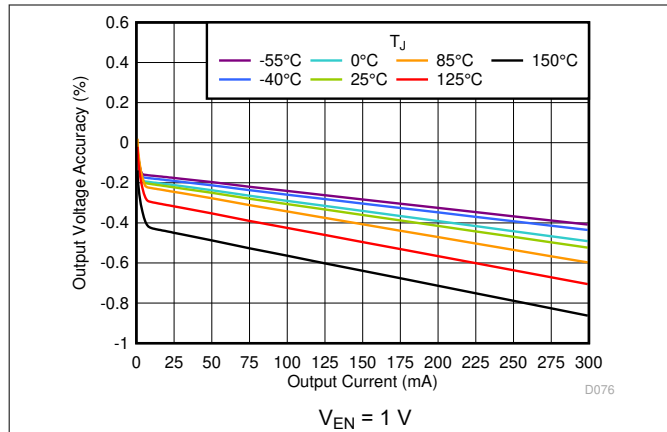
图 5-7. Output Voltage Accuracy vs I_{OUT}
