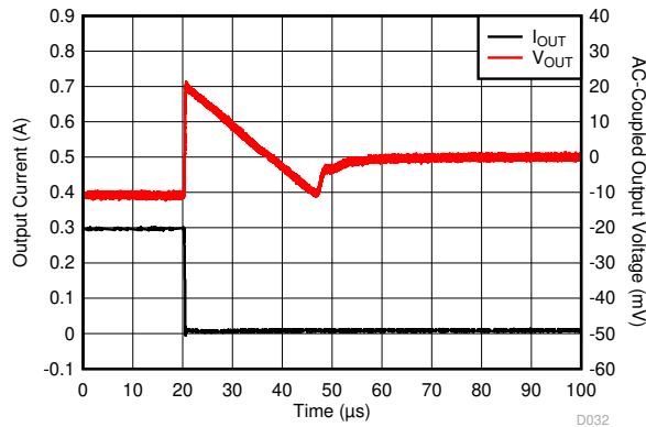
图 5-37. Load Transient
