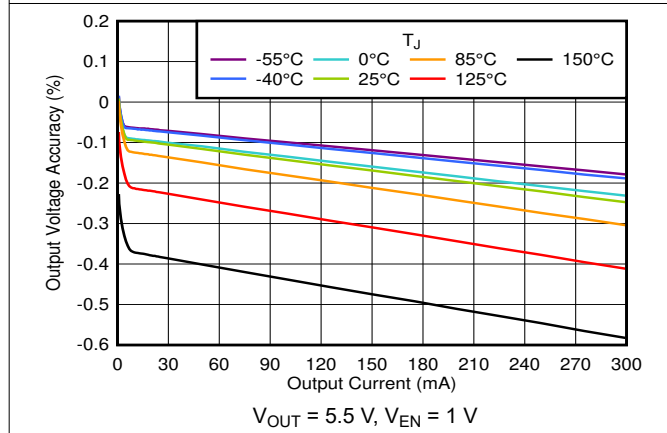
图 5-9. Output Voltage Accuracy vs I_{OUT}
