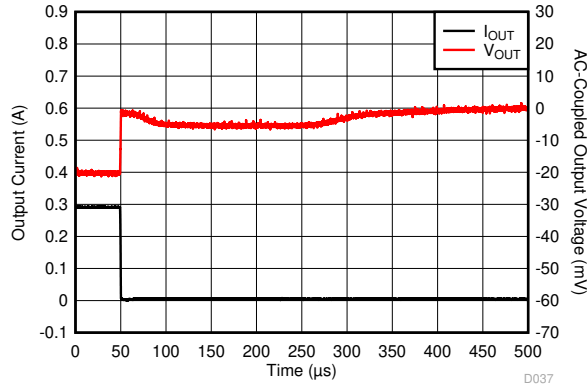
图 5-37. Load Transient
