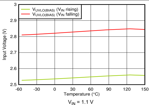
7-63. V_{BIAS} UVLO vs Temperature
