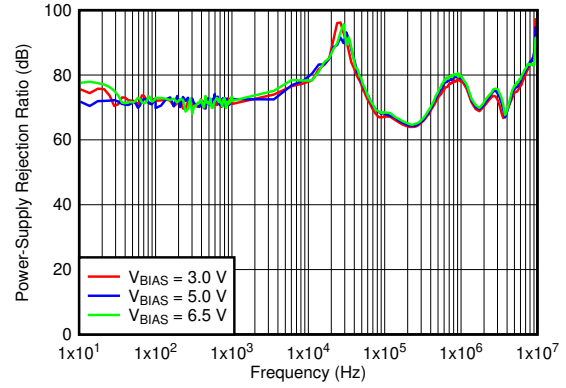
7-8. V_{BIAS} PSRR vs Frequency
