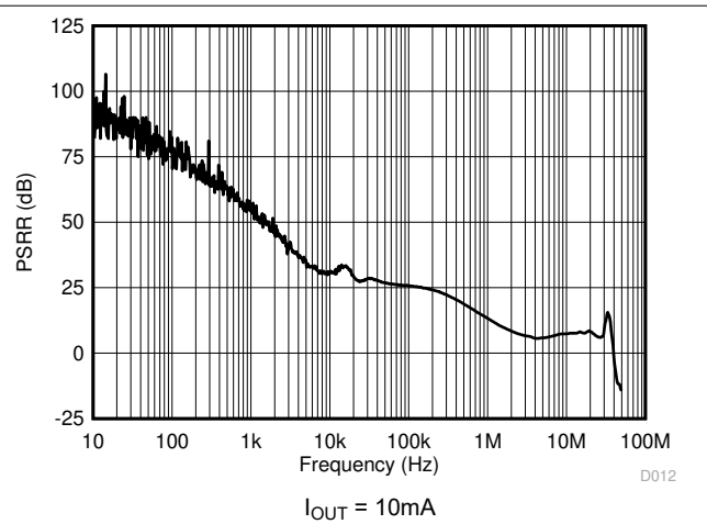
図 5-12. PSRR と周波数との関係
