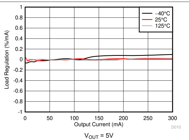
図 5-10. 負荷の制御
