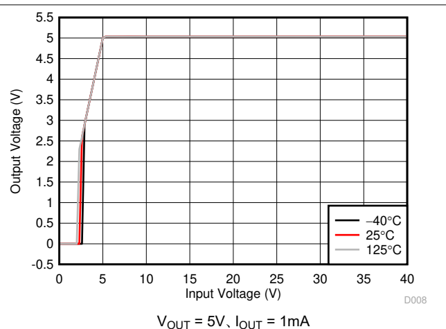
図 5-8. 出力電圧と入力電圧との関係
