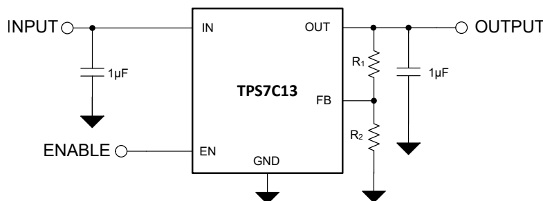
図 7-1. TPS7C13 の代表的なアプリケーション
