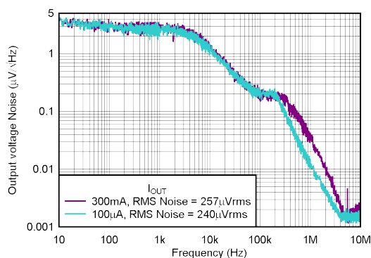
図 5-17. ノイズ
