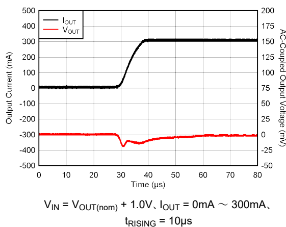
図 5-11. 負荷過渡
