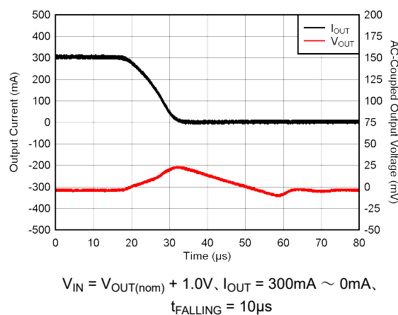
図 5-12. 負荷過渡
