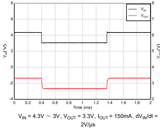
図 5-47. ドロップアウトからの回復 (4.3V 入力 3V 出力)
