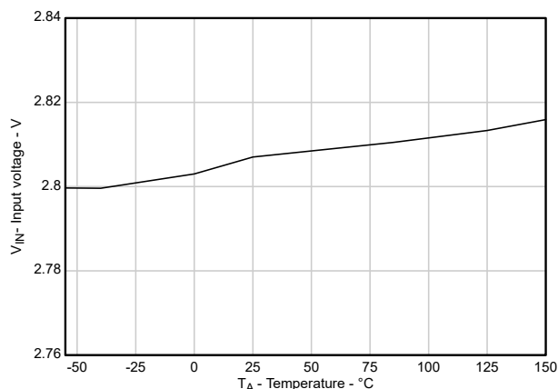
図 5-18. UVLO 立ち上がりスレッショルド ( V_{UVLO+} ) と温度との関係
