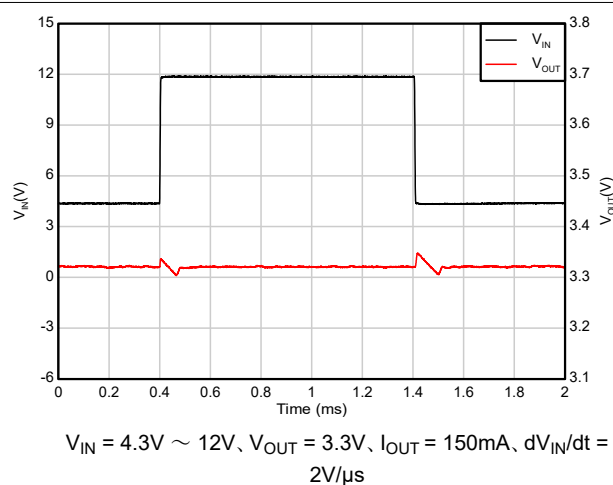
図 5-41. ライン過渡応答 (4.3V ~ 12V)
