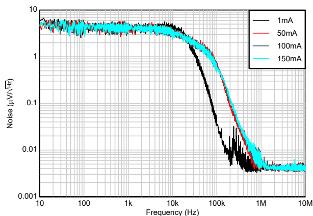
図 5-25. ノイズと I_{OUT} との関係
