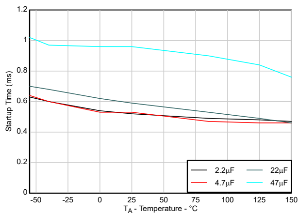
図 5-20. スタートアップタイムと C_{OUT} との関係
