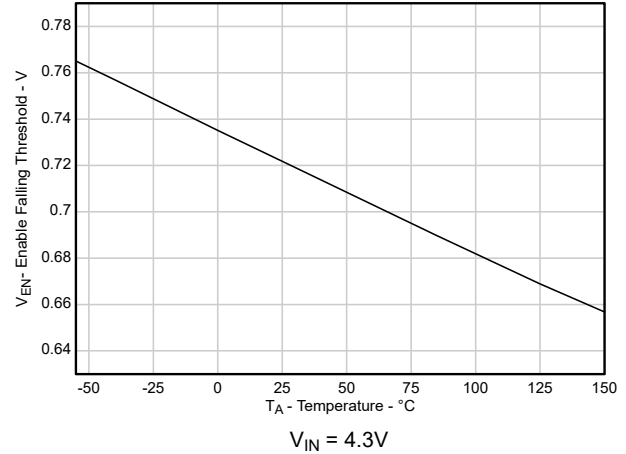
図 5-14. EN 立ち下がりスレッショルド V_{IL(EN)} と温度との関係
