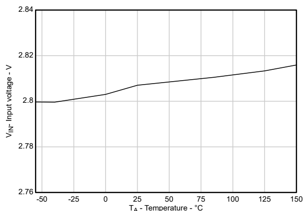
図 5-19. UVLO 立ち下がりスレッショルド ( V_{UVLO-} ) と温度との関係
