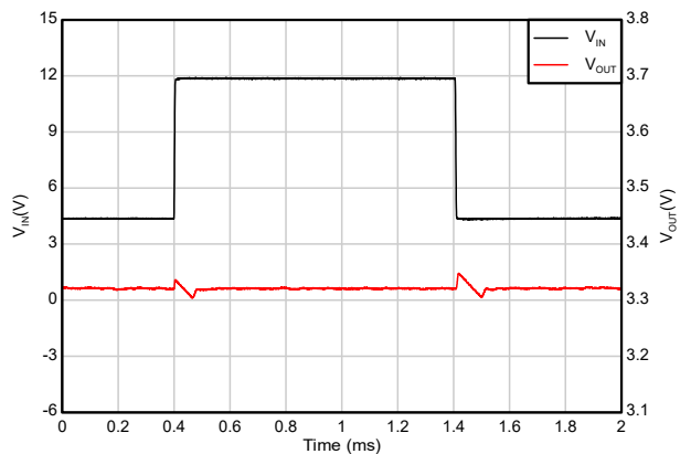
図 7-11. ライン過渡応答 (4.3V ~ 12V)
