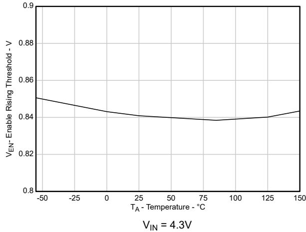
図 5-13. EN 立ち上がりスレッショルド V_{IH(EN)} と温度との関係
