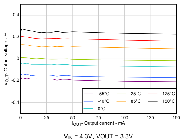
図 2-1. V_{\text{OUT}} の精度と I_{\text{OUT}} との関係
