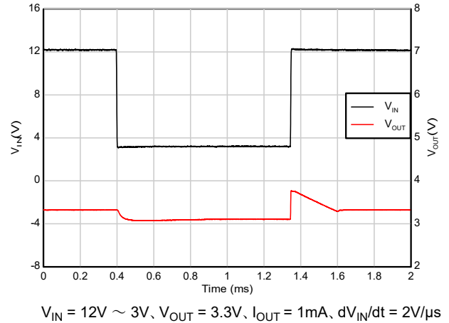
図 5-48. ドロップアウトからの回復 (12V 入力 3V 出力)
