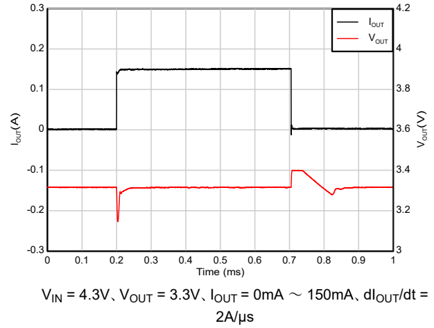
図 5-44. 負荷過渡応答 (0mA~150mA)
