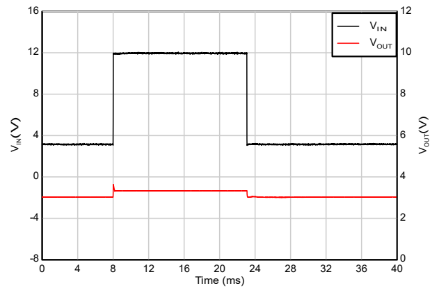
図 5-50. コールドクランク回復
