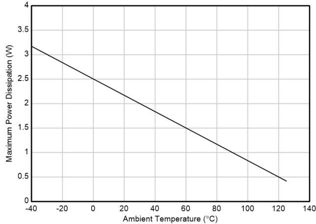
図 7-4. TPS7E81-Q1 (DGN) 許容消費電力
