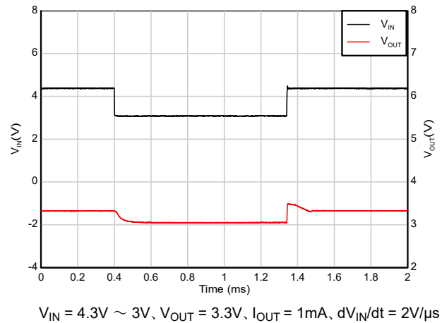
図 5-46. ドロップアウトからの回復 (4.3V 入力 3V 出力)
