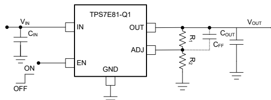
図 3-1. 代表的なアプリケーション
