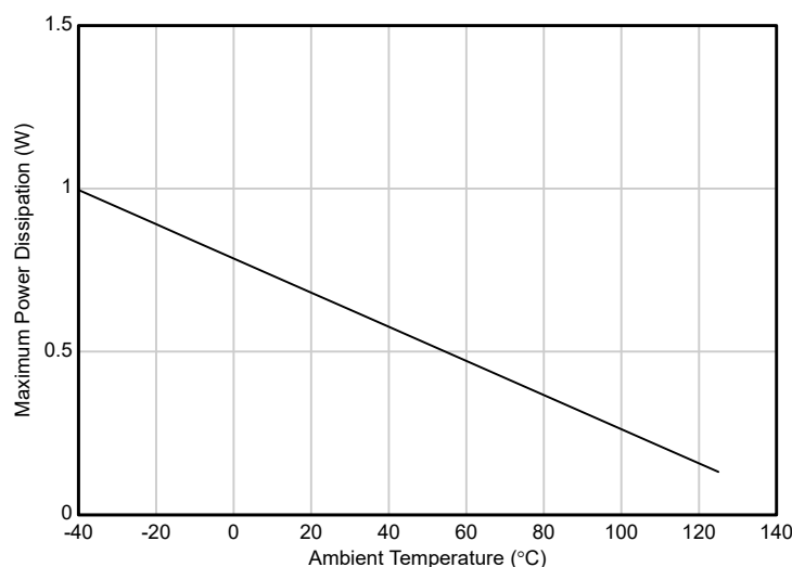
図 7-2. TPS7E81-Q1 (DBV) 許容消費電力
