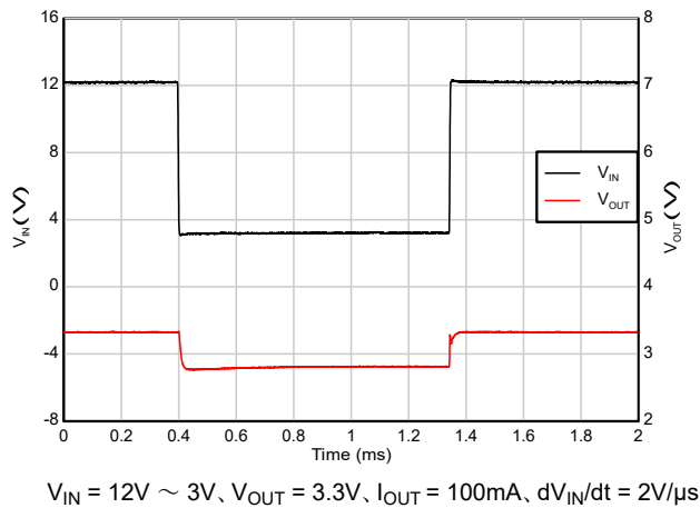
図 5-49. ドロップアウトからの回復 (12V 入力 3V 出力)
