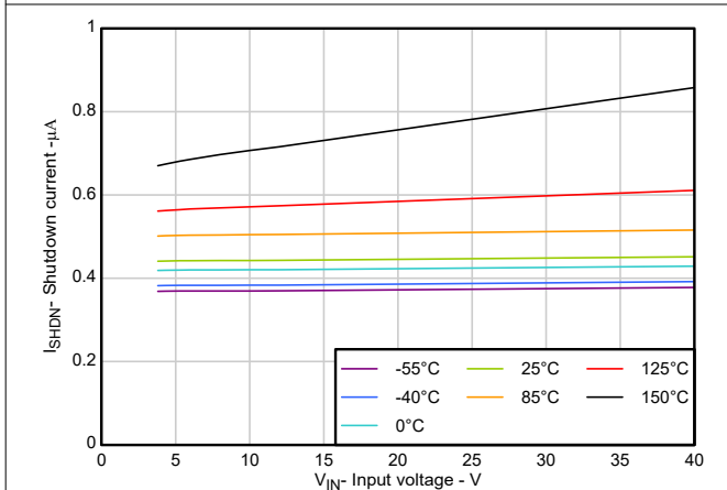
図 5-11. I_{SHDN} と V_{IN} との関係
