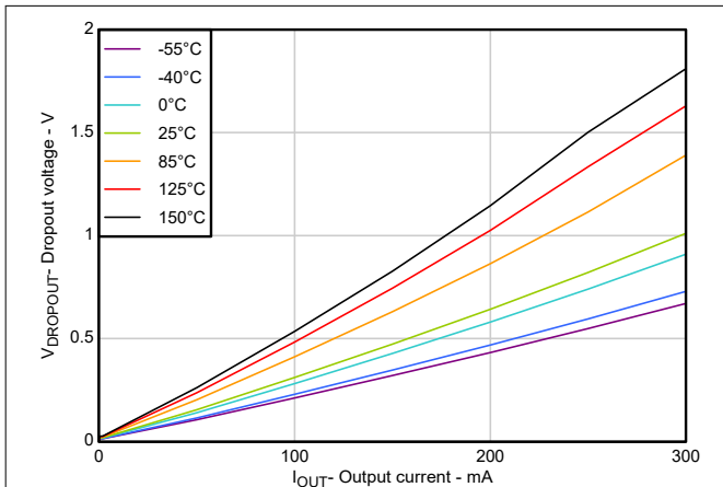
図 5-7. V_{DO} と I_{OUT}(\text{mA}) との関係
