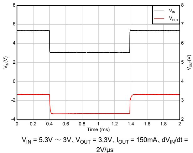
図 5-44. ドロップアウトからの回復 (5.3V 入力 3V 出力)
