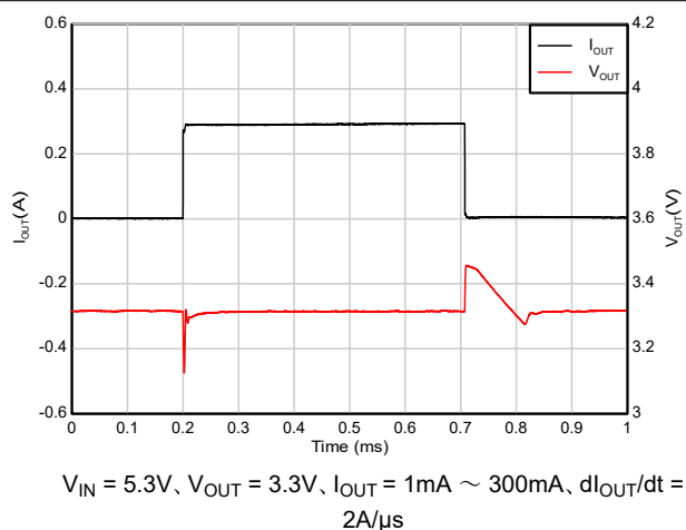
図 7-13. 負荷過渡応答 (1mA~300mA)
