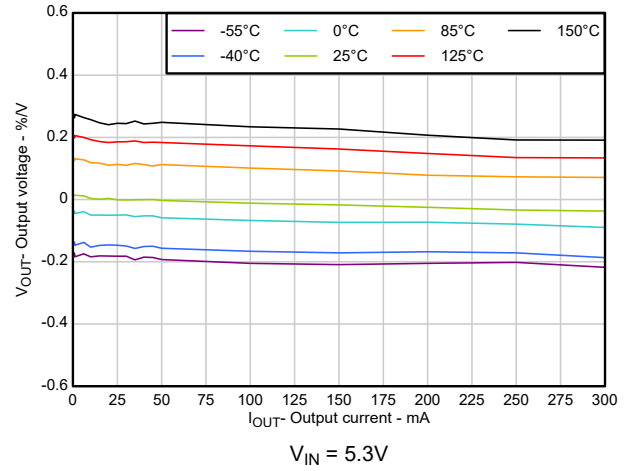
図 5-2. V_{OUT} の精度と I_{OUT} との関係
