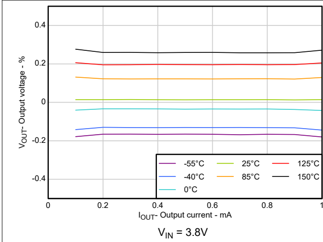
図 5-1. V_{OUT} の精度と I_{OUT} との関係
