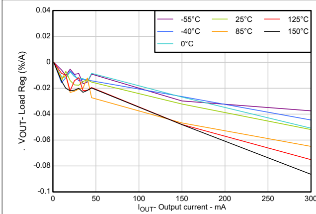
図 5-5. ロードレギュレーション
