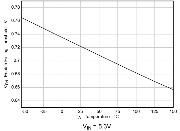
図 5-14. EN 立ち下がりスレッシュヨルド V_{IL(EN)} と温度との関係
