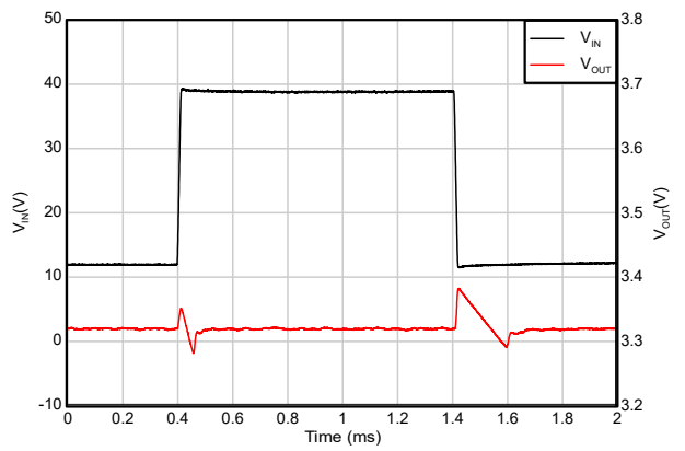
図 5-39. ライン過渡応答 (12V ~ 40V)
