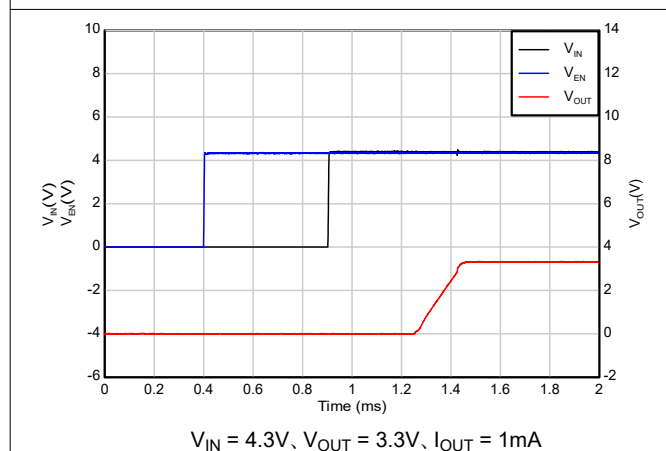
図 5-35. シーケンスによる起動 (EN 後ろの V_{IN} )
