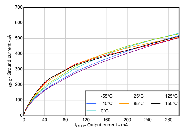
図 5-10. I_{GND} と I_{OUT} との関係
