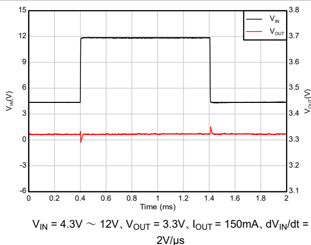
図 7-11. ライン過渡応答 (4.3V ~ 12V)
