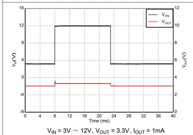
図 5-47. コールドクランク回復
