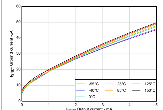
図 5-9. I_{GND} と I_{OUT} との関係
