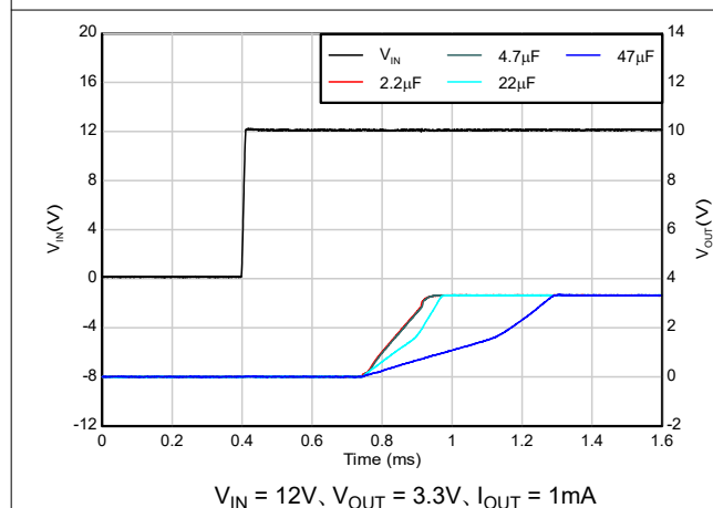
図 5-29. スタートアップと C_{OUT} との関係
