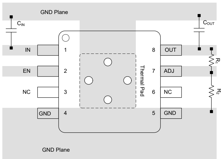
図 7-21. TPS7E82-Q1 DGN パッケージのレイアウト例
