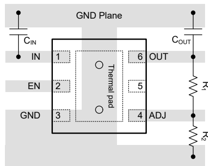
図 7-20. TPS7E82-Q1 DRV パッケージのレイアウト例
