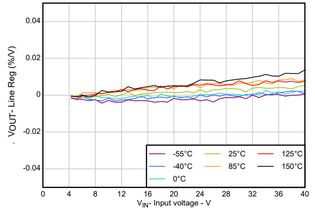
図 5-4. ラインレギュレーション
