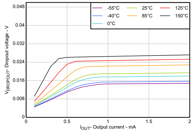
図 5-6. V_{DO} と I_{OUT}(\text{mA}) との関係
