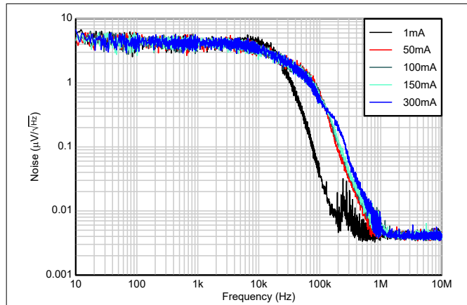
図 5-25. ノイズと I_{OUT} との関係
