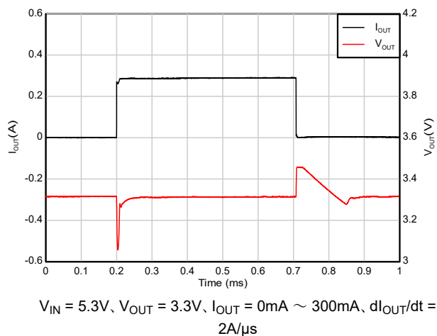
図 5-41. 負荷過渡応答 (0mA~300mA)
