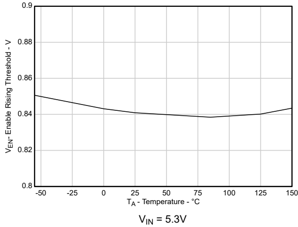
図 5-13. EN 立ち上がりスレッシュヨルド V_{IH(EN)} と温度との関係
