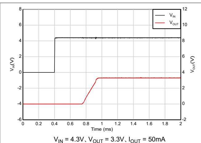
図 5-32. EN & V_{IN} を互いに接続した状態でのスタートアップ
