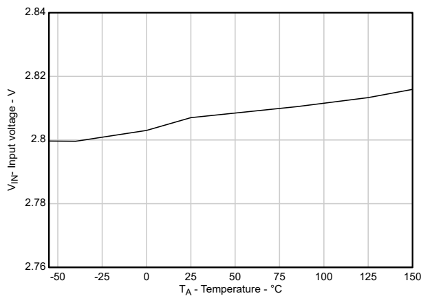
図 5-19. UVLO 立ち下がりスレッショルド ( V_{\text{UVLO-}} ) と温度との関係
