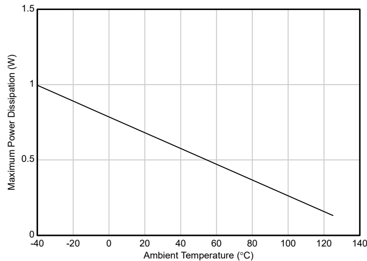
図 7-2. TPS7E82-Q1 (DBV) 許容消費電力
