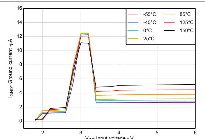
図 5-8. I_{GND} と V_{IN} との関係
