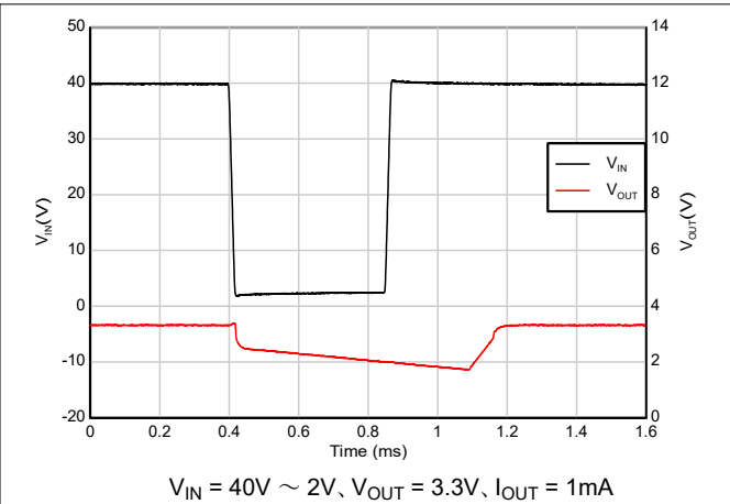
図 7-16. ブラウンアウトからの回復 (40V ~ 2V)
