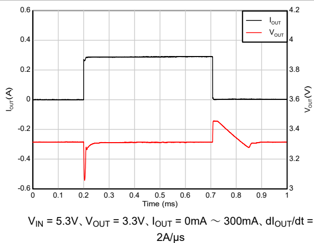
図 7-12. 負荷過渡応答 (0mA~300mA)
