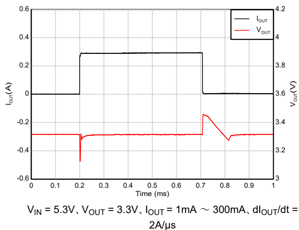
図 5-42. 負荷過渡応答 (1mA~300mA)
