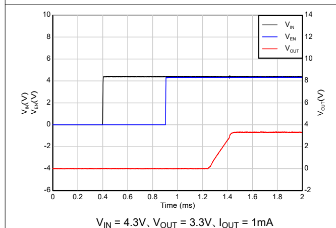
図 5-33. シーケンスによる起動 ( V_{IN} 後の EN)
