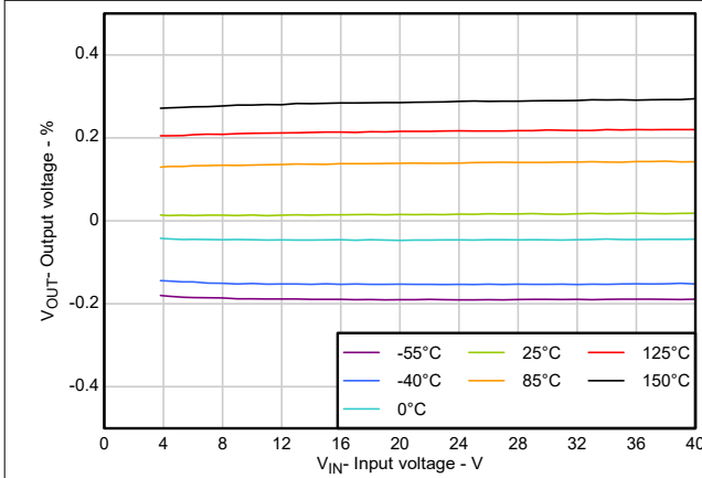
図 5-3. V_{OUT} の精度と V_{IN} との関係
