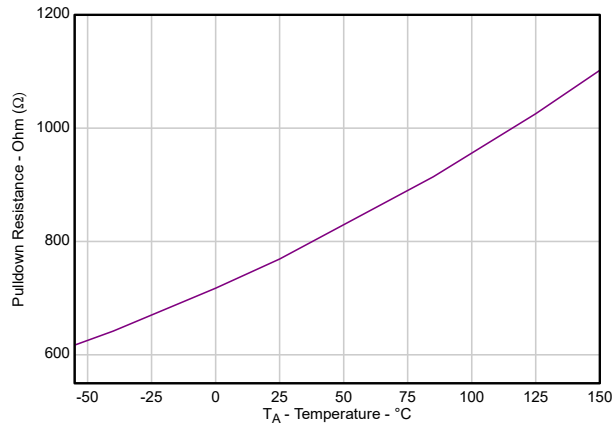
図 5-17. 出力のプルダウン抵抗 ( R_{\text{Discharge}} ) と温度との関係
