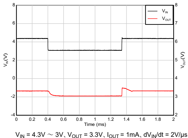
図 5-43. ドロップアウトからの回復 (4.3V 入力 3V 出力)
