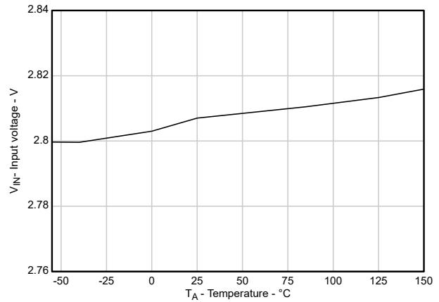
図 5-18. UVLO 立ち上がりスレッショルド ( V_{\text{UVLO+}} ) と温度との関係
