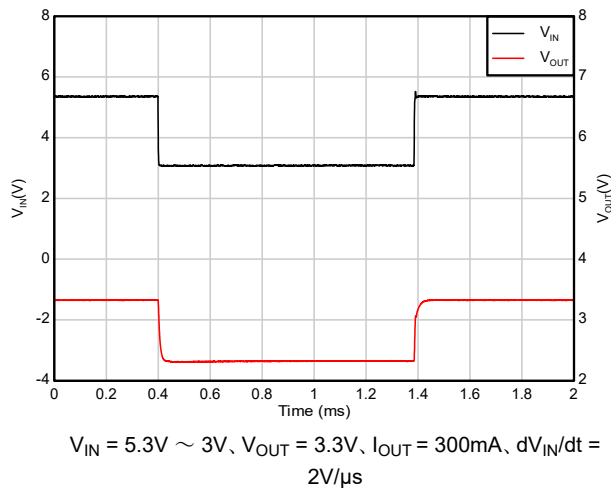
図 7-15. ドロップアウトからの回復 (5.3V 入力 3V 出力)
