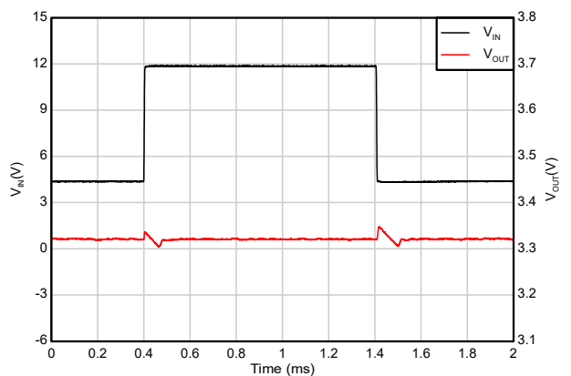
図 5-37. ライン過渡応答 (4.3V ~ 12V)
