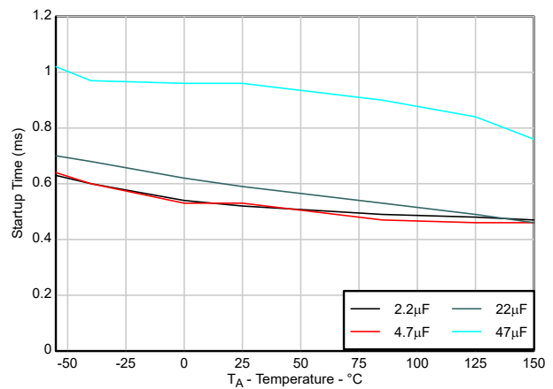
図 5-20. スタートアップタイムと C_{\text{OUT}} との関係
