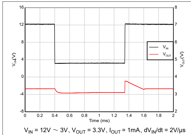
図 5-45. ドロップアウトからの回復 (12V 入力 3V 出力)
