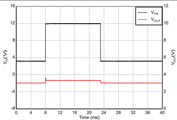
図 5-45. ドロップアウトからの回復 (12V 入力 3V 出力)
