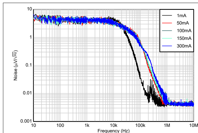
図 5-25. ノイズと I_{OUT} との関係
