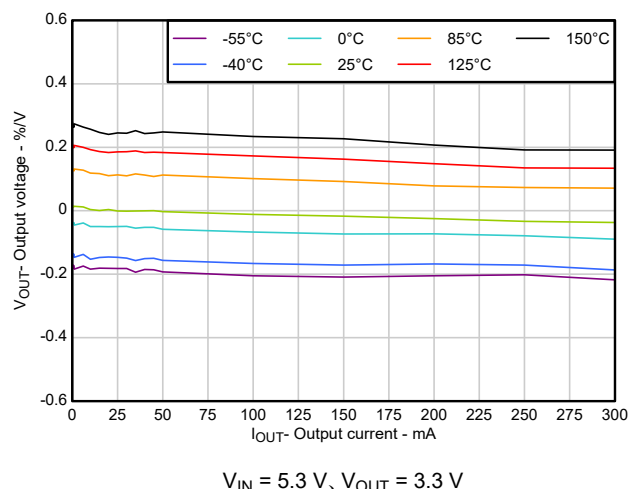
図 2-1. V_{\text{OUT}} の精度と I_{\text{OUT}} との関係
