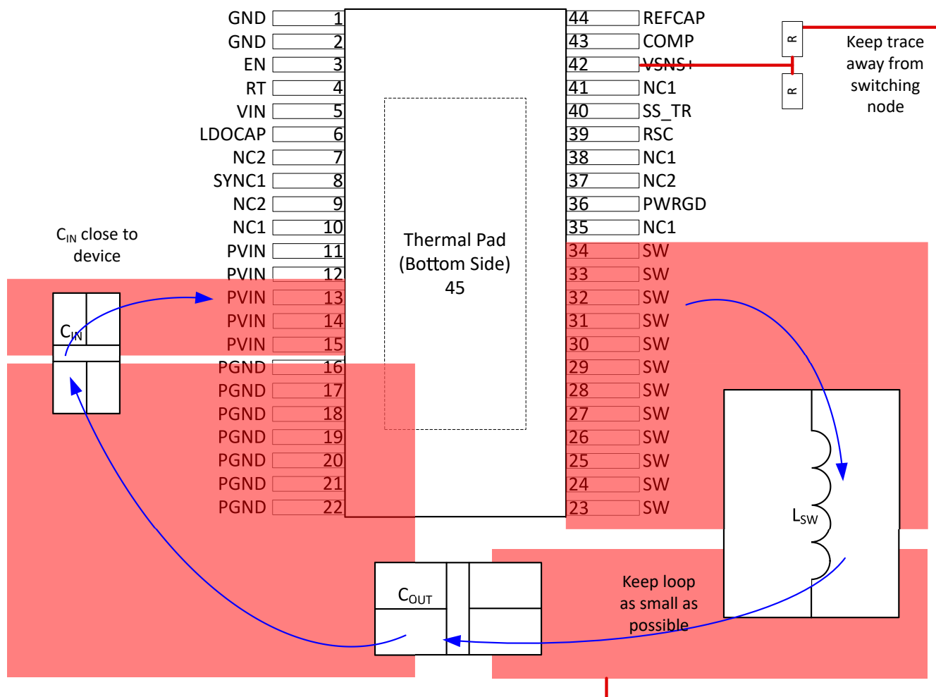
図 10-5. 簡略化されたレイアウト例
