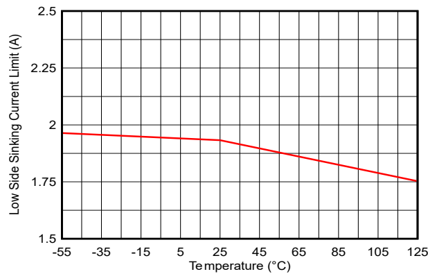
図 7-39. ローサイドシンク電流制限スレッショルド (I OC_LS(sink) ) と温度との関係
