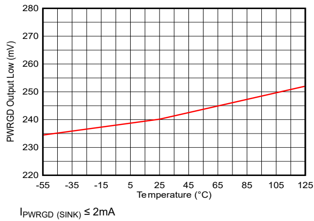
図 7-51. パワーグッド出力 Low と温度との関係
