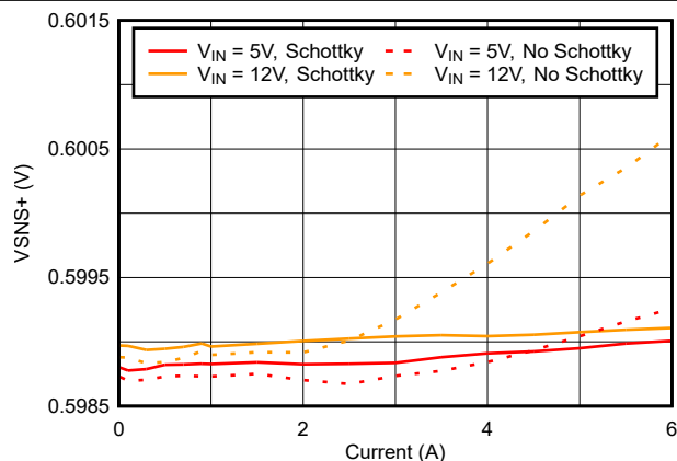
図 7-32. 1MHz での VSNS+ と出力電流の関係
