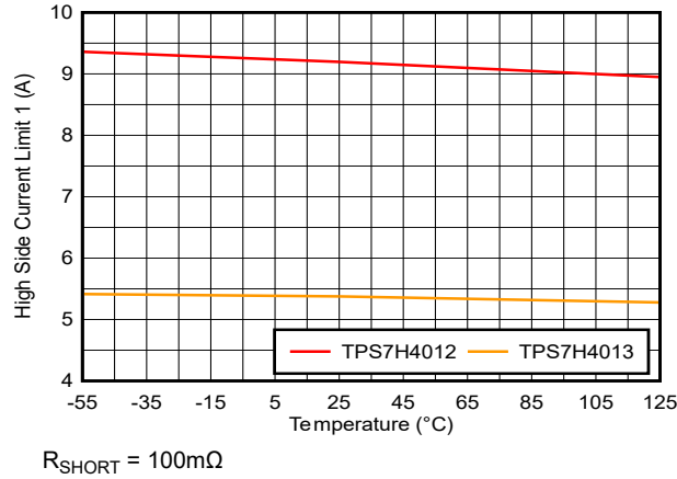
図 7-37. ハイサイド電流制限スレッショルド 1 (I OC_HS1 ) と温度との関係
