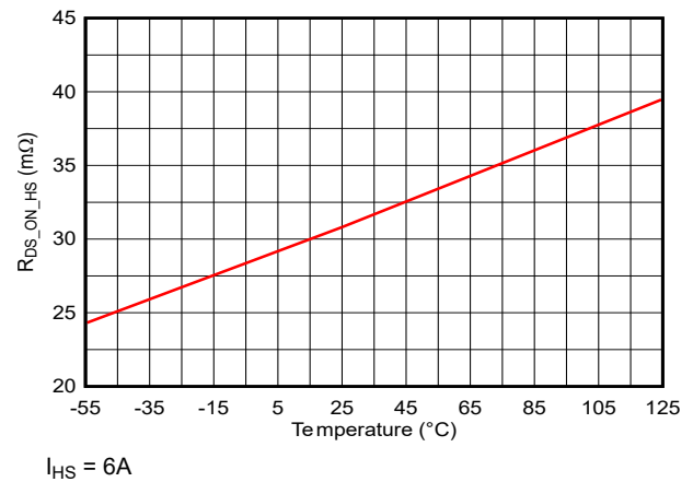
図 7-52. ハイサイド FET 抵抗と温度との関係
