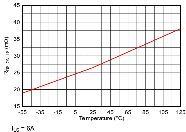
図 7-53. ローサイド FET 抵抗と温度との関係
