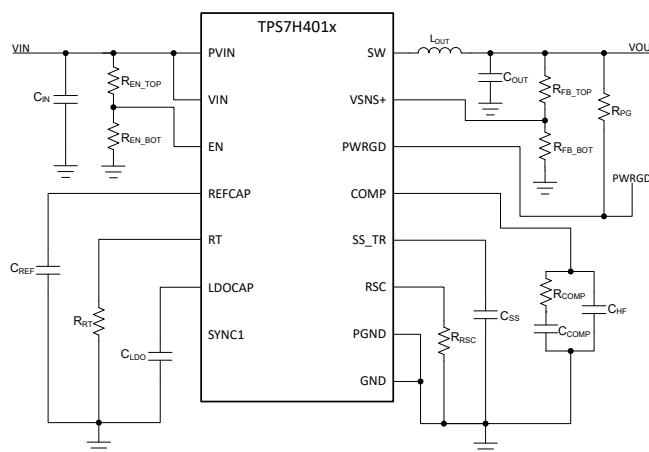
概略回路図
