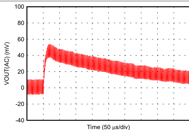
図 7-55. 立ち下がり負荷ステップ: 226A/μs で 5.5A から 0A まで
