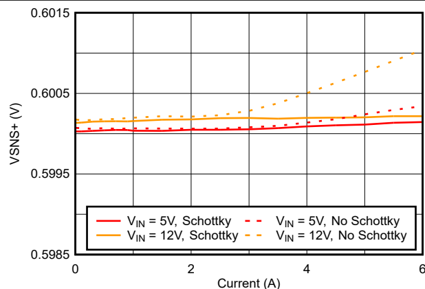
図 7-31. 500kHz での VSNS+ と出力電流の関係
