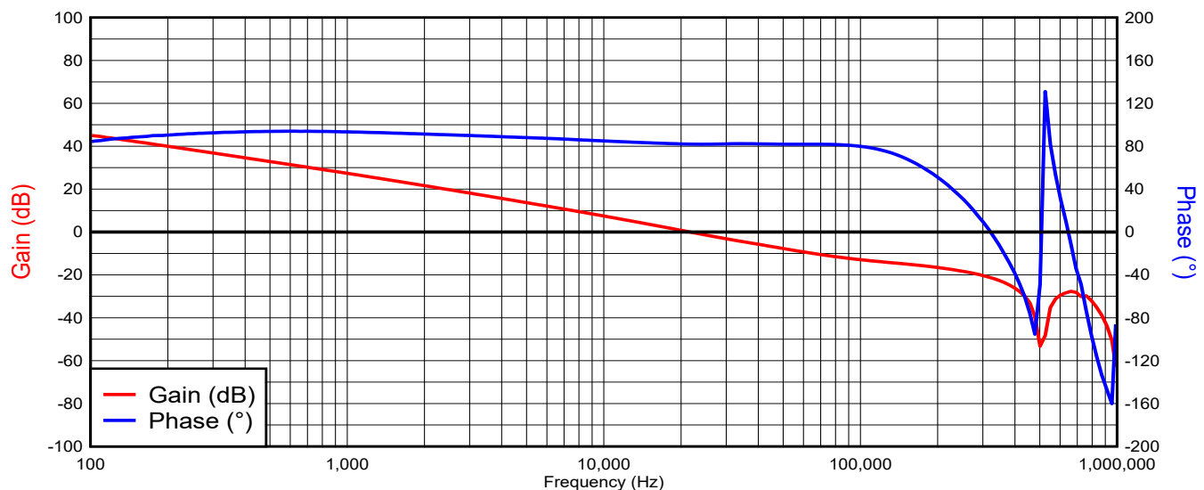
図 10-3. ボード線図
