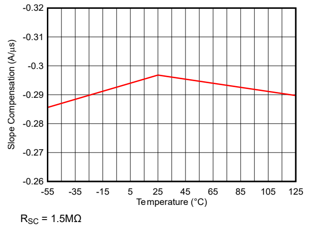
図 7-40. スロープ補償と温度との関係 (100kHz 時)
