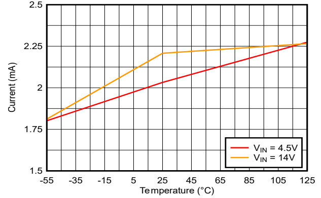
図 7-26. V_{IN} シャットダウン電流と温度との関係
