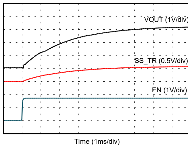
図 7-56. スタートアップ
