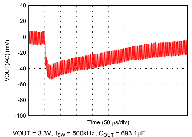
図 7-54. 立ち上がり負荷ステップ: 203A/μs で 0A から 5.5A まで
