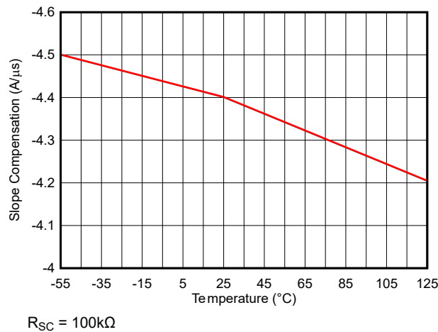
図 7-41. スロープ補償と温度との関係 (500kHz 時)
