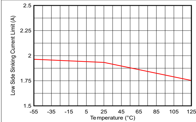
図 7-39. ローサイドシンク電流制限スレッシュヨルド ( I_{OC\_LS(sink)} ) と温度との関係
