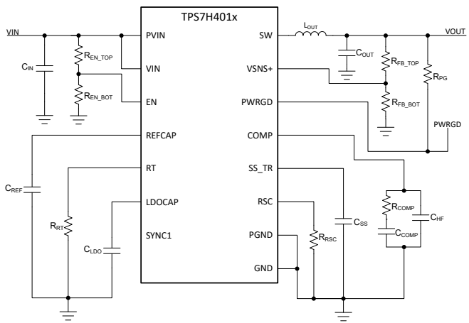
概略回路図
