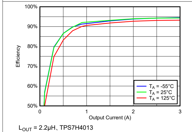
図 7-23. 温度全体に対する効率と負荷との関係 (500kHz、VIN = 12V、VOUT = 5V、TPS7H4013)
