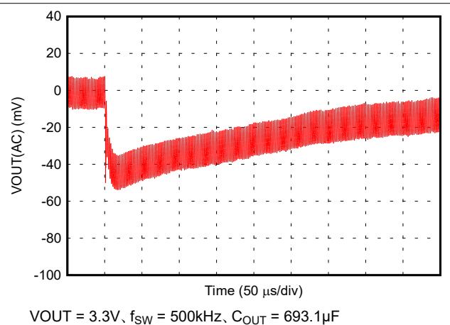
図 7-54. 立ち上がり負荷ステップ: 203A/μs で 0A から 5.5A まで
