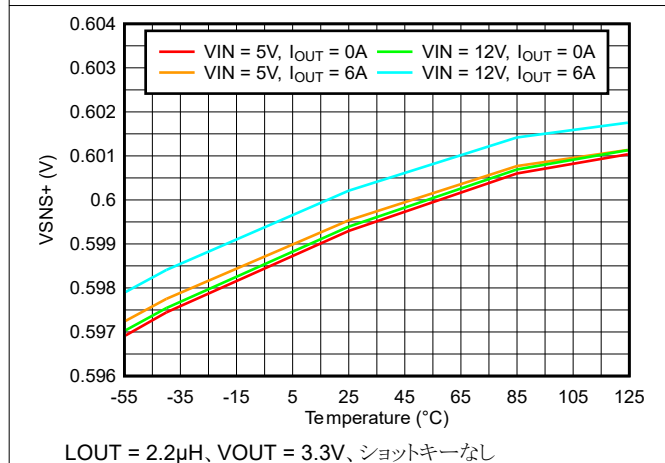
図 7-33. 500kHz での VSNS+ と温度との関係
