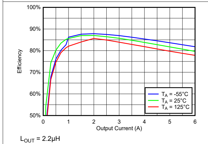
図 7-15. 温度全体に対する効率と負荷との関係 (500kHz、VIN = 5V、VOUT = 1.1V)
