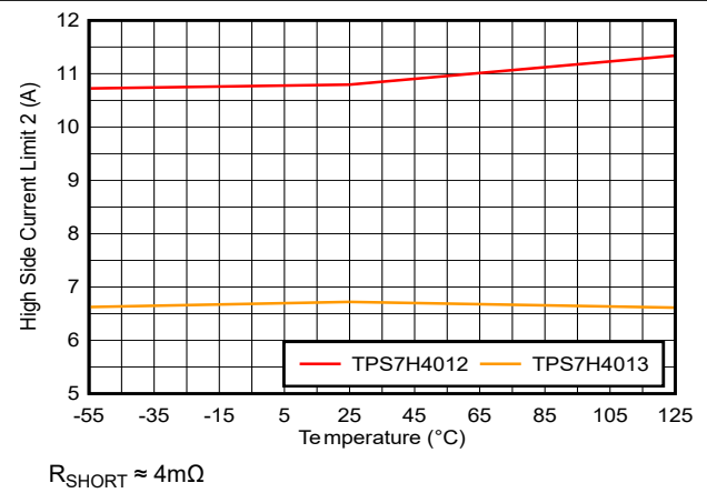
図 7-38. ハイサイド電流制限スレッシュヨルド 2 ( I_{OC\_HS2} ) と温度との関係
