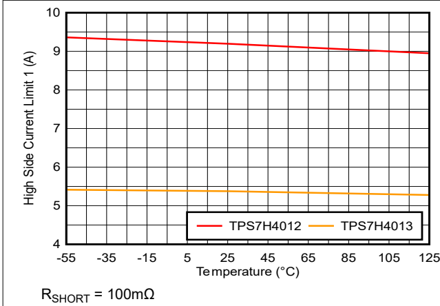
図 7-37. ハイサイド電流制限スレッシュヨルド 1 ( I_{OC\_HS1} ) と温度との関係
