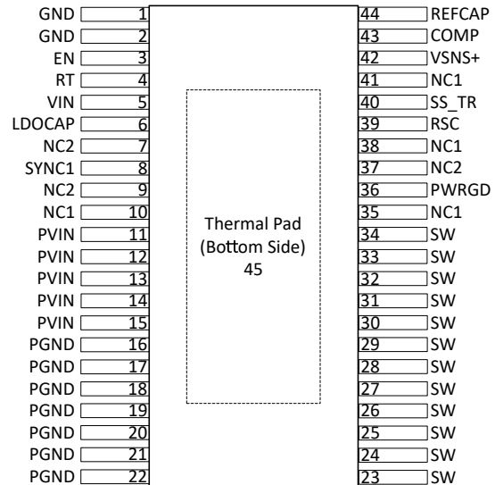
図 6-2. DDW パッケージ、44 ピン HTSSOP (上面図)
