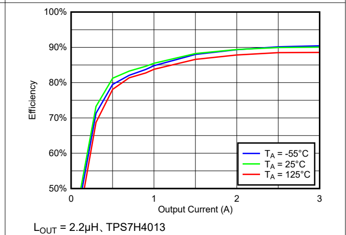
図 7-24. 温度全体に対する効率と負荷との関係 (500kHz、VIN = 12V、VOUT = 2.5V、TPS7H4013)
