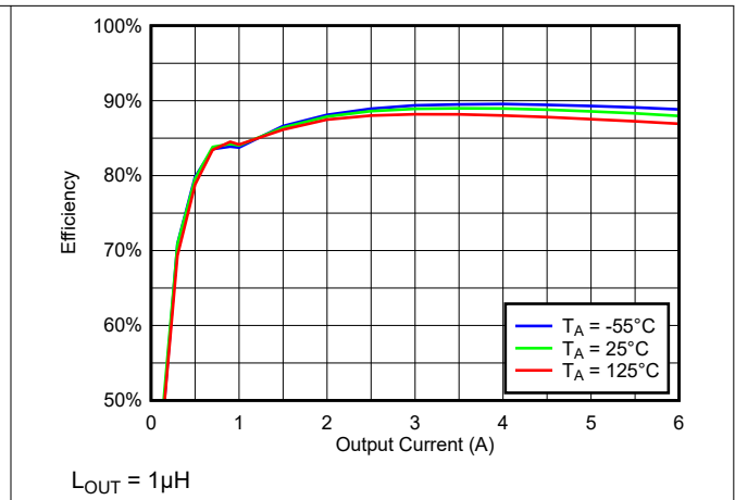
図 7-22. 温度全体に対する効率と負荷との関係 (1MHz、VIN = 12V、VOUT = 3.3V)
