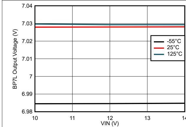
7-15. BP7L Output Voltage vs VIN Voltage
