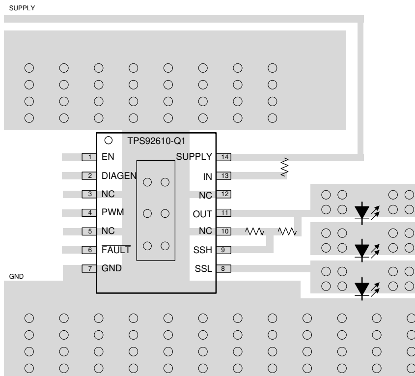
☒ 27. TPS92610-Q1 Example Layout Diagram
