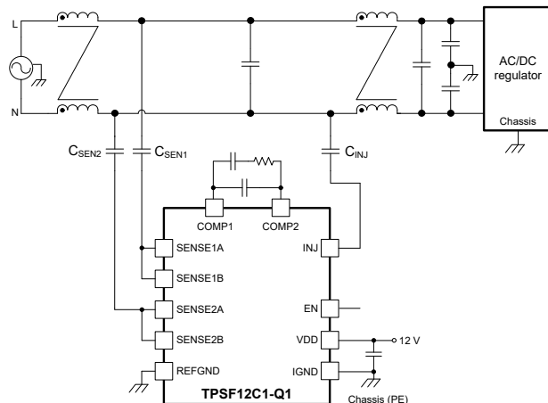
簡略回路図
