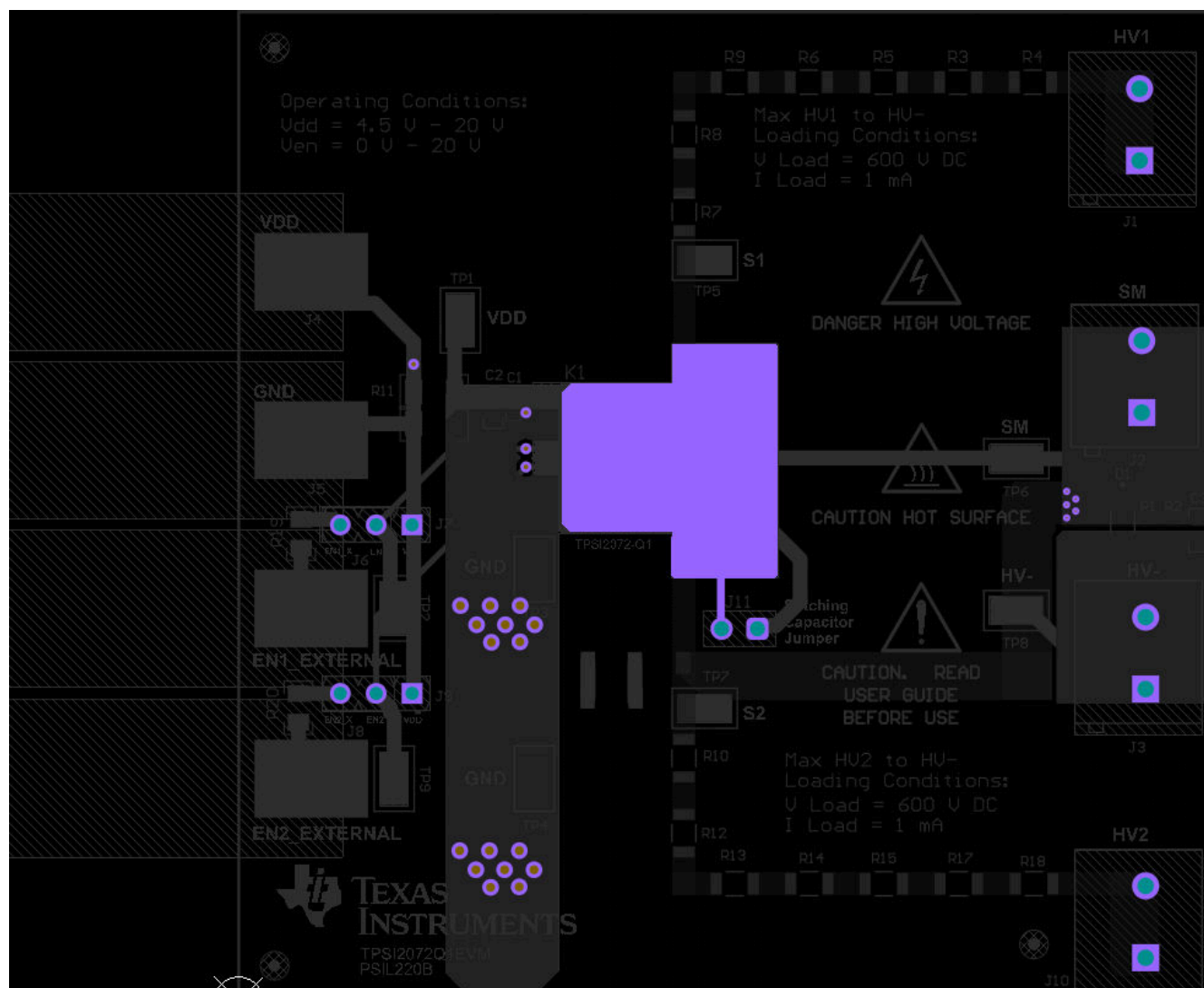
9-17. TPSI2072-Q1 EVM - Layer 5
