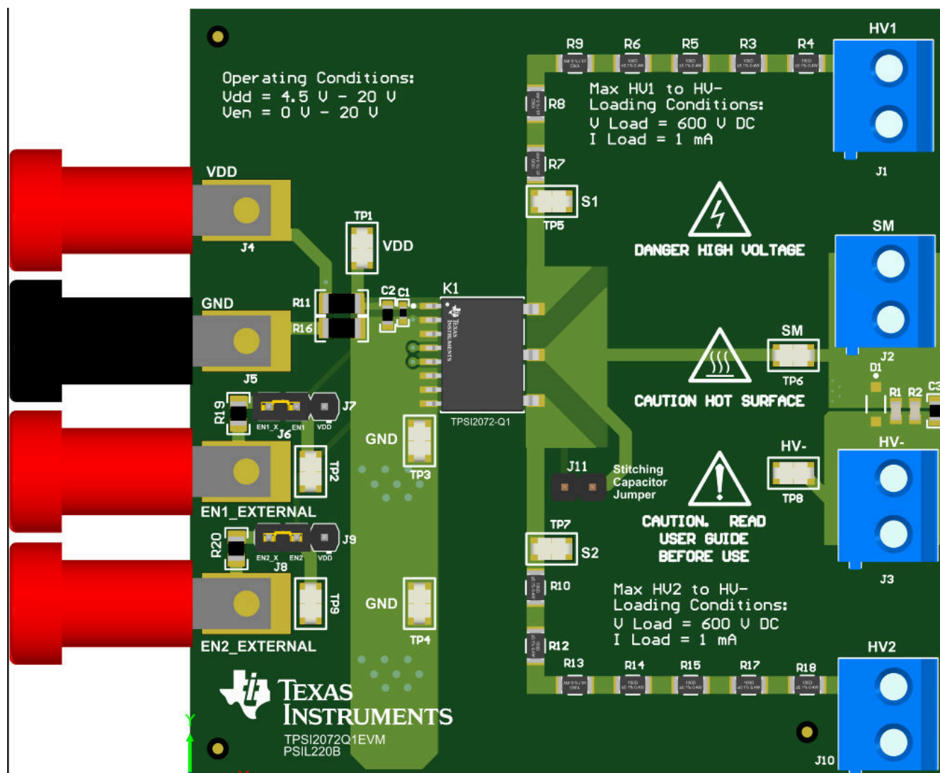
図 9-12. TPSI2072-Q1 EVM - Component View
