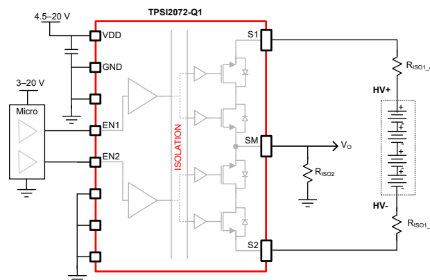
TPSI2072-Q1 アプリケーション概略回路図
