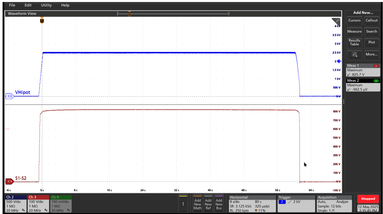
図 9-9. V HIPOT = 2500V でのアバランシェ電圧 (s1-s2) (900kΩ の制限抵抗を使用)
