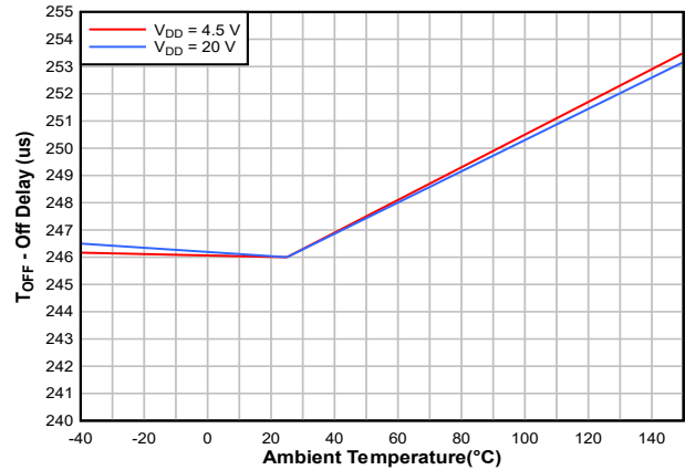
図 6-8. 入力から出力オフまでの遅延 ( V_{IN} = 500V )
