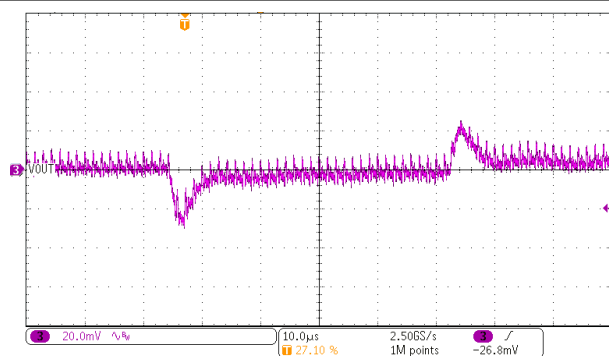
8-4. 10-A Transient Load Step
