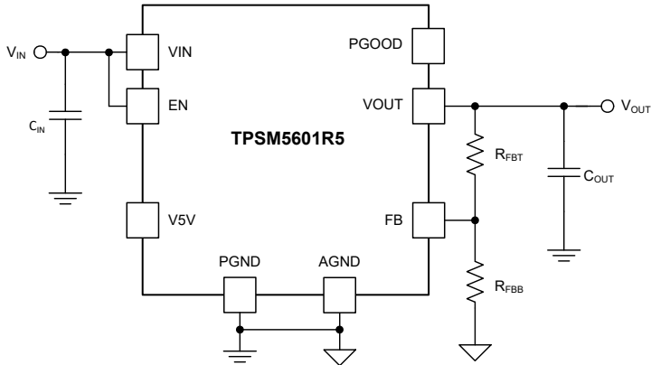
代表的な回路図
