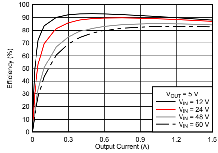
標準的な効率、 V_{OUT} = 5V
